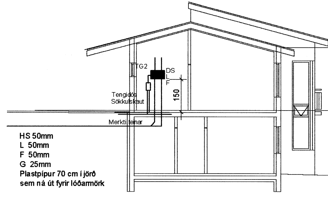
Sökkulskaut mkv. 1:100
