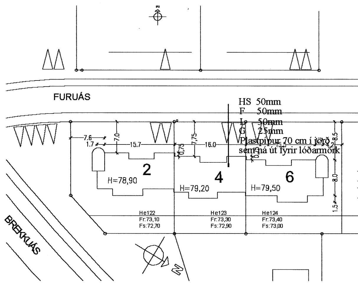
Afstöðumynd mkv. 1:500
