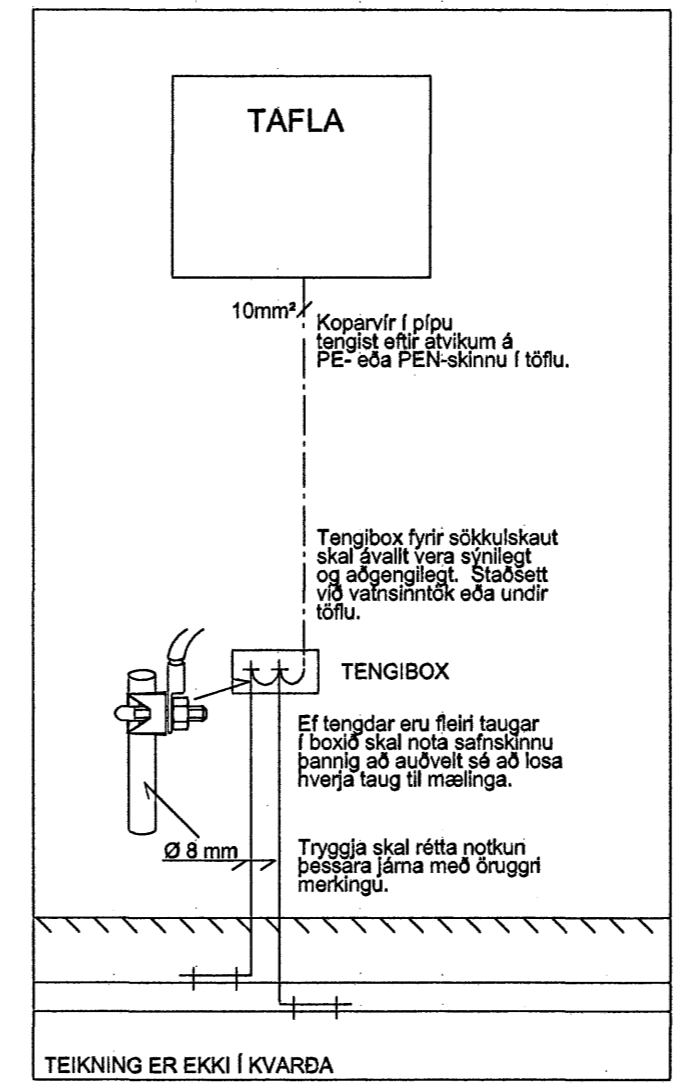
SNID Í TÖFLUVEGG DÆMIGERÐUR FRÁGANGUR
