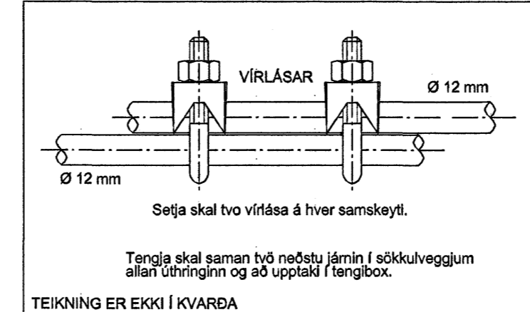
SAMTENGING STEYPUPEINA DÆMIGERÐUR FRÁGANGUR
