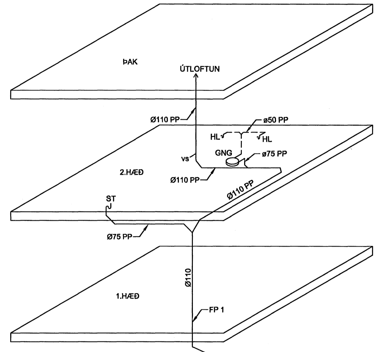
RÚMMYND STAMMA MKV. 1:50
