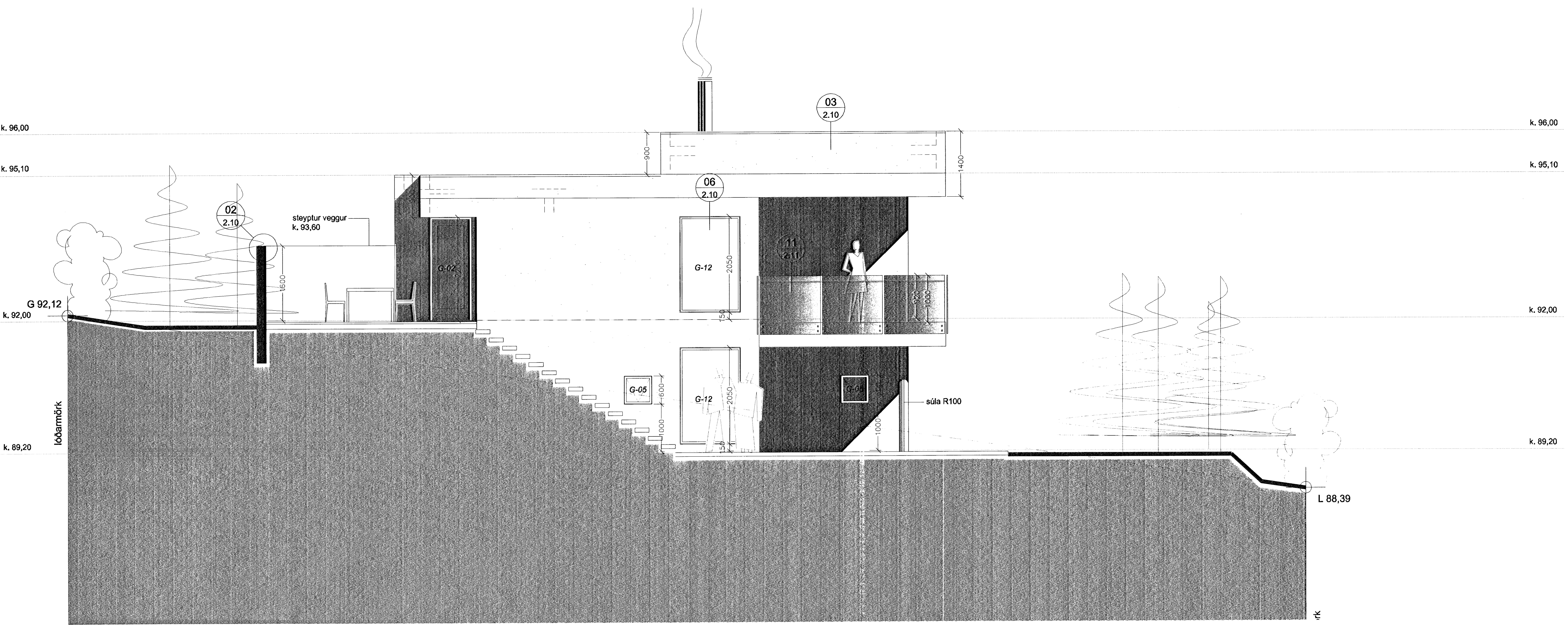
ÚTLIT SUÐUR M 1 : 50
