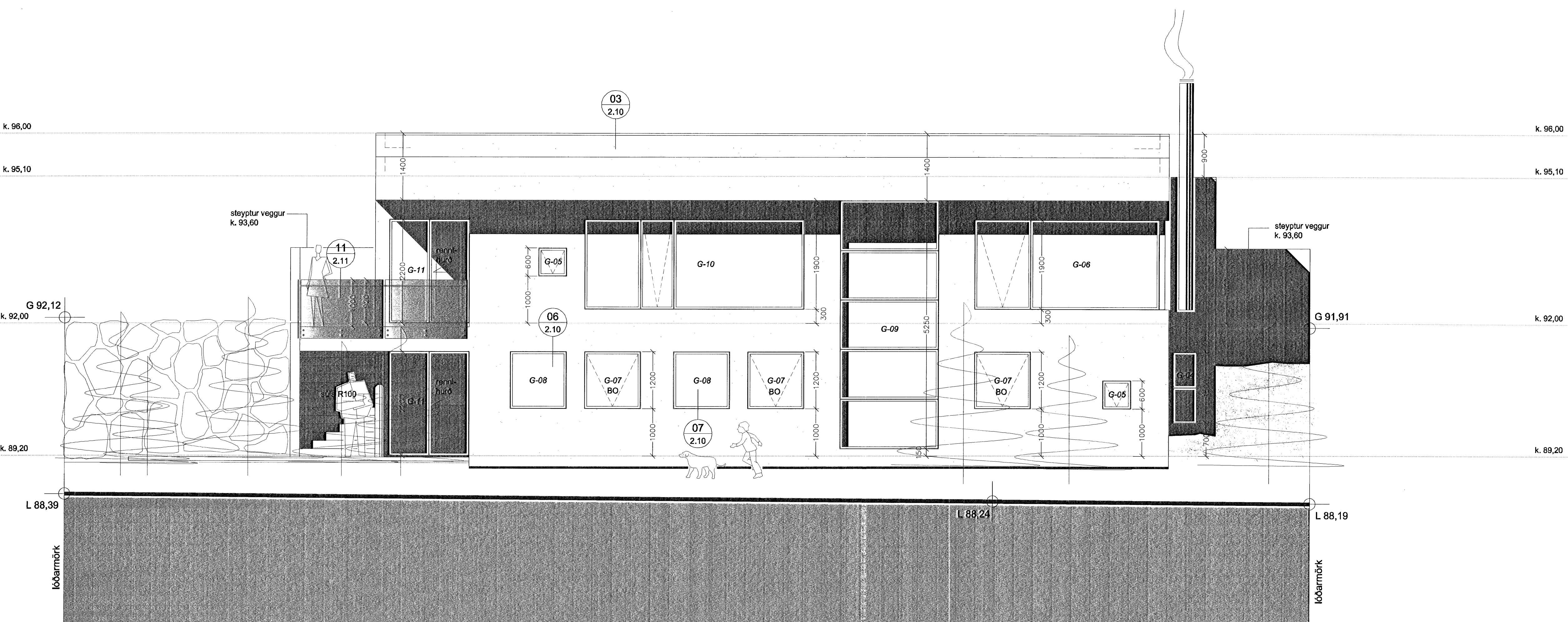
ÚTLIT AUSTUR M 1 : 50
