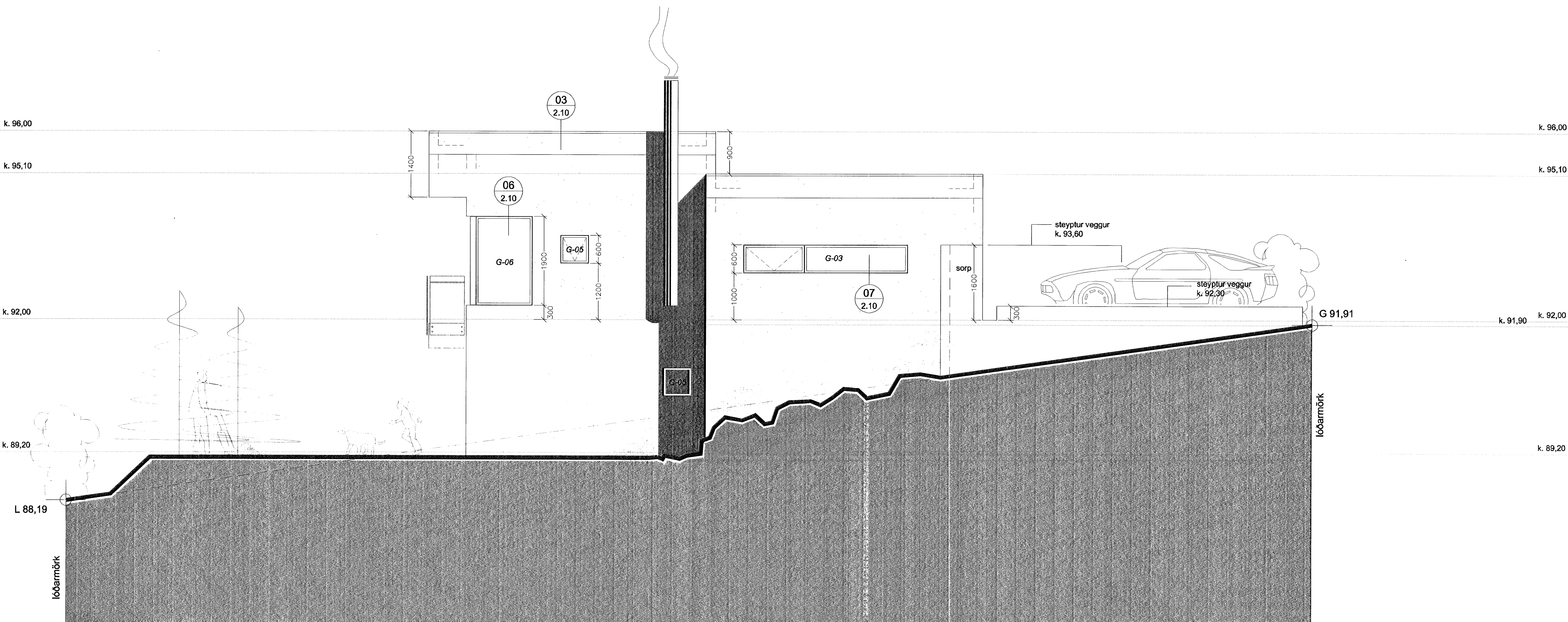
ÚTLIT NORÐUR M 1 : 50
