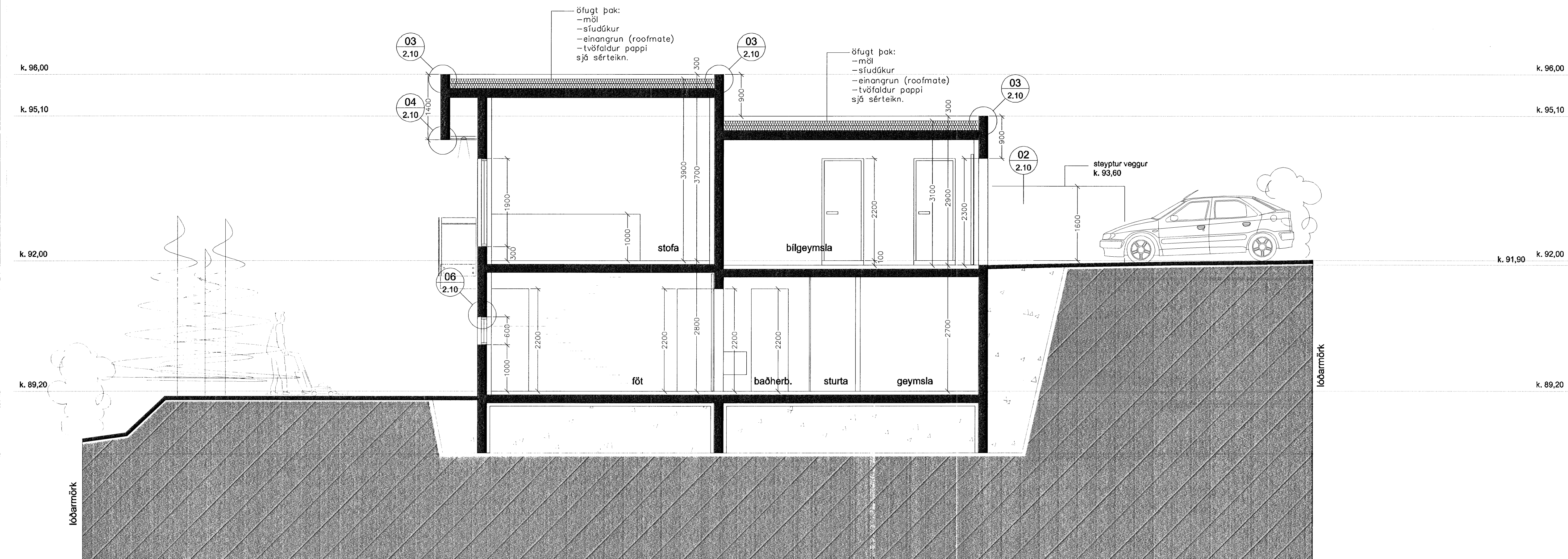
SNEIÐING C - C M 1 : 50
