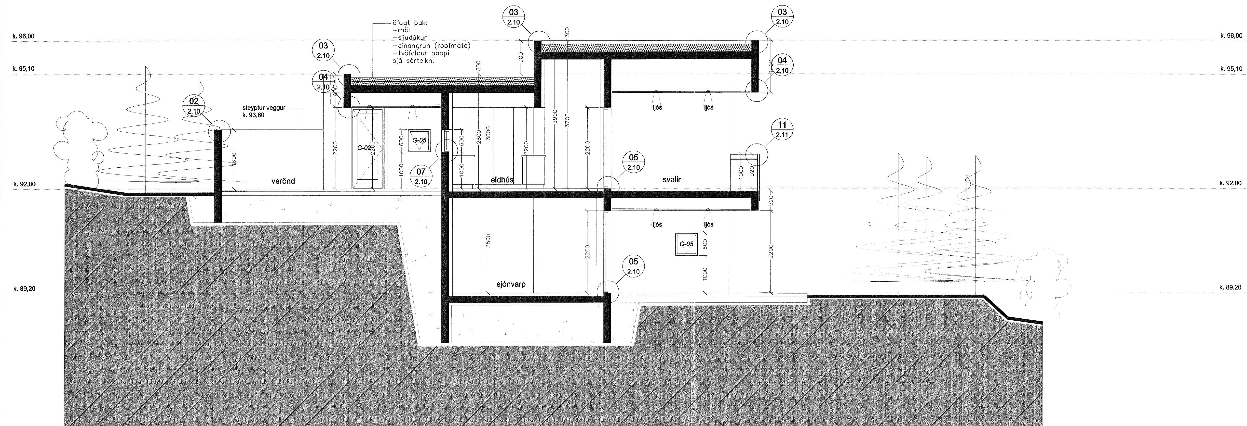
SNEIÐING D - D M 1 : 50
