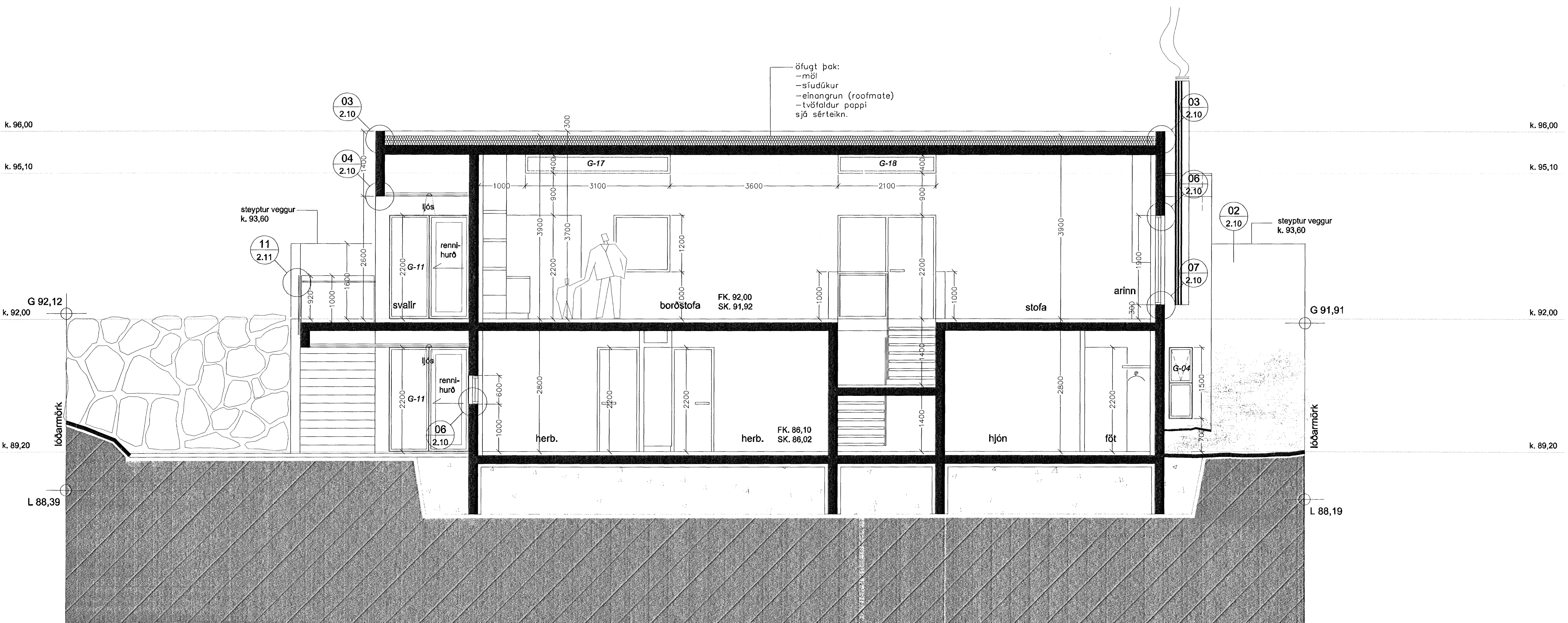
SNEIDING B - B M 1 : 50
