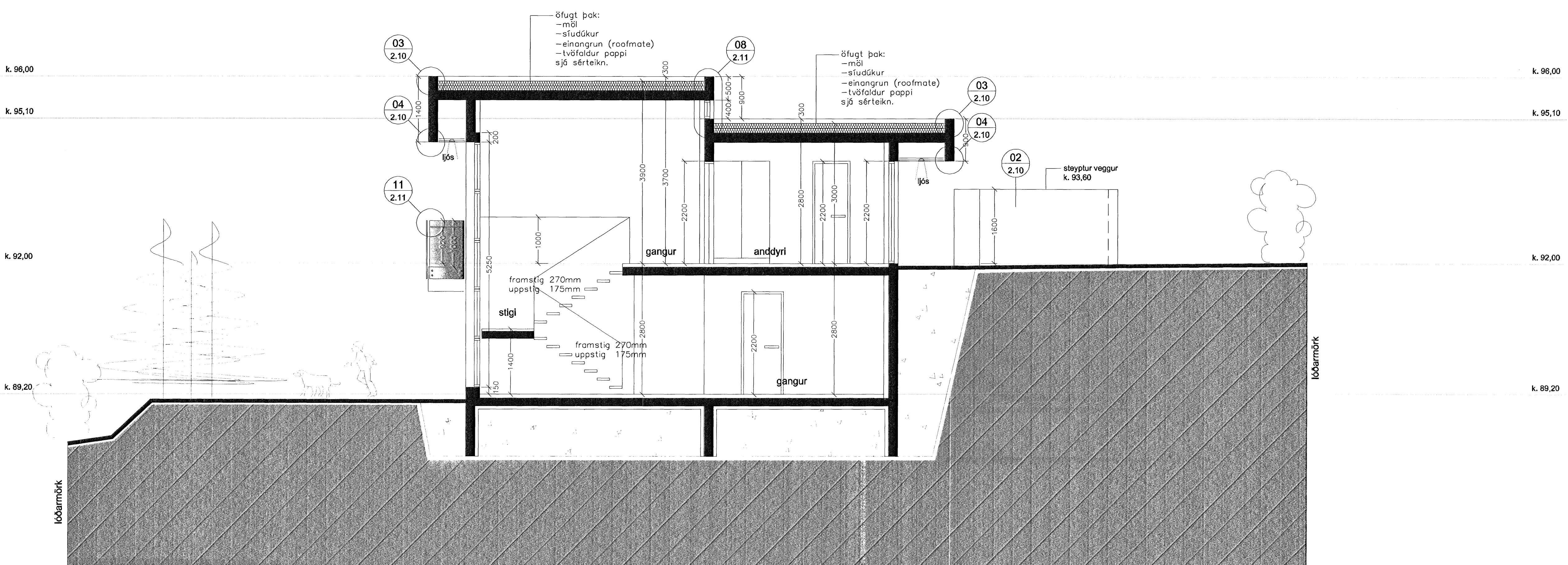
SNEIDING A - A M 1 : 50
