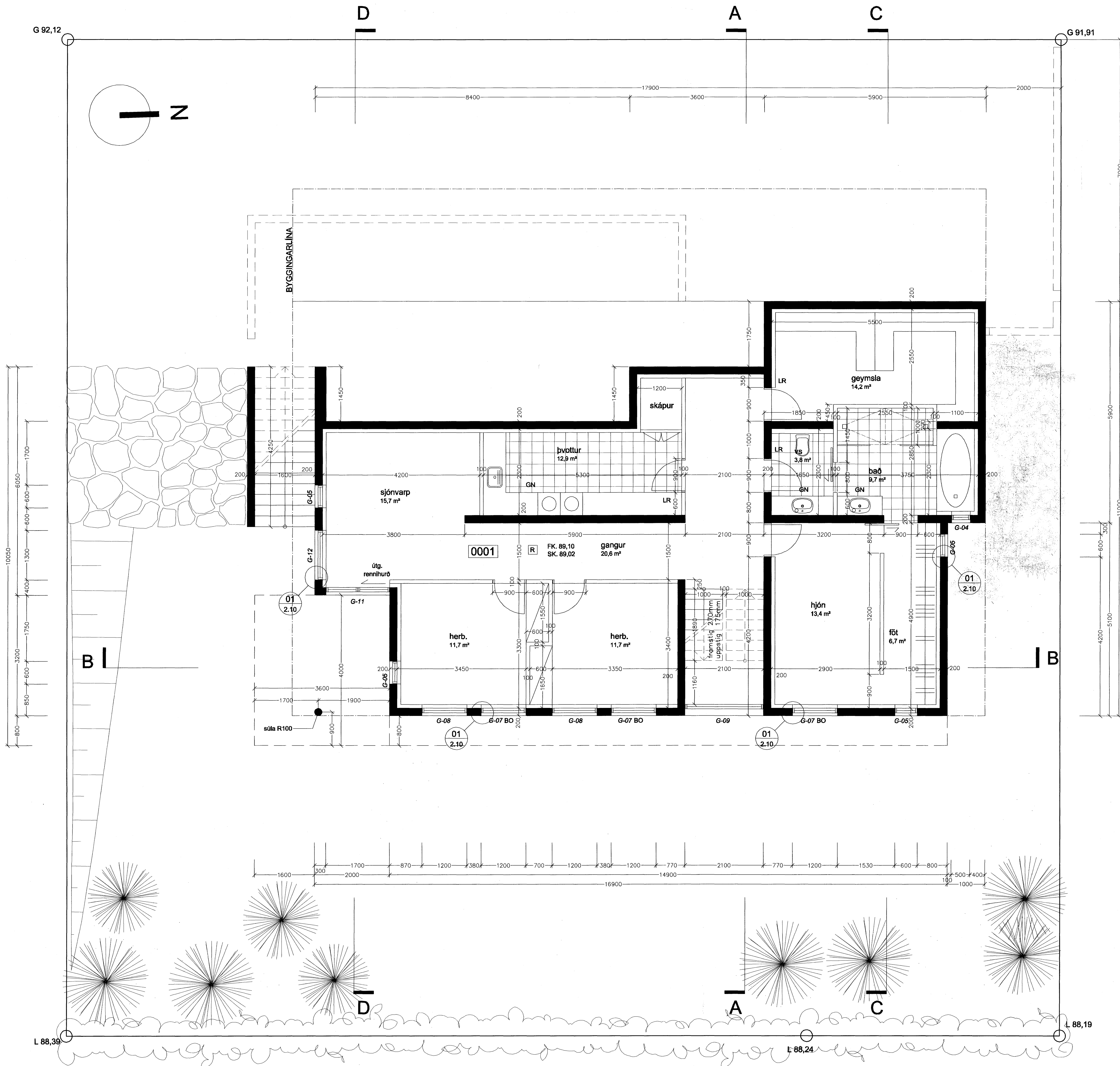
GRUNNMYND NEDRI HÆÐ M 1 : 50
