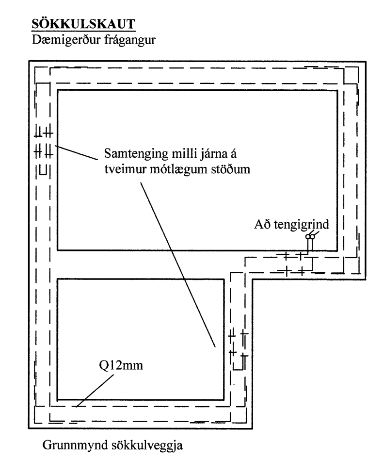
FRÁGANGUR Á SAMTENGINGUM STEYPUSTEINA FYRIR SÖKKULJARÐSKAUT
