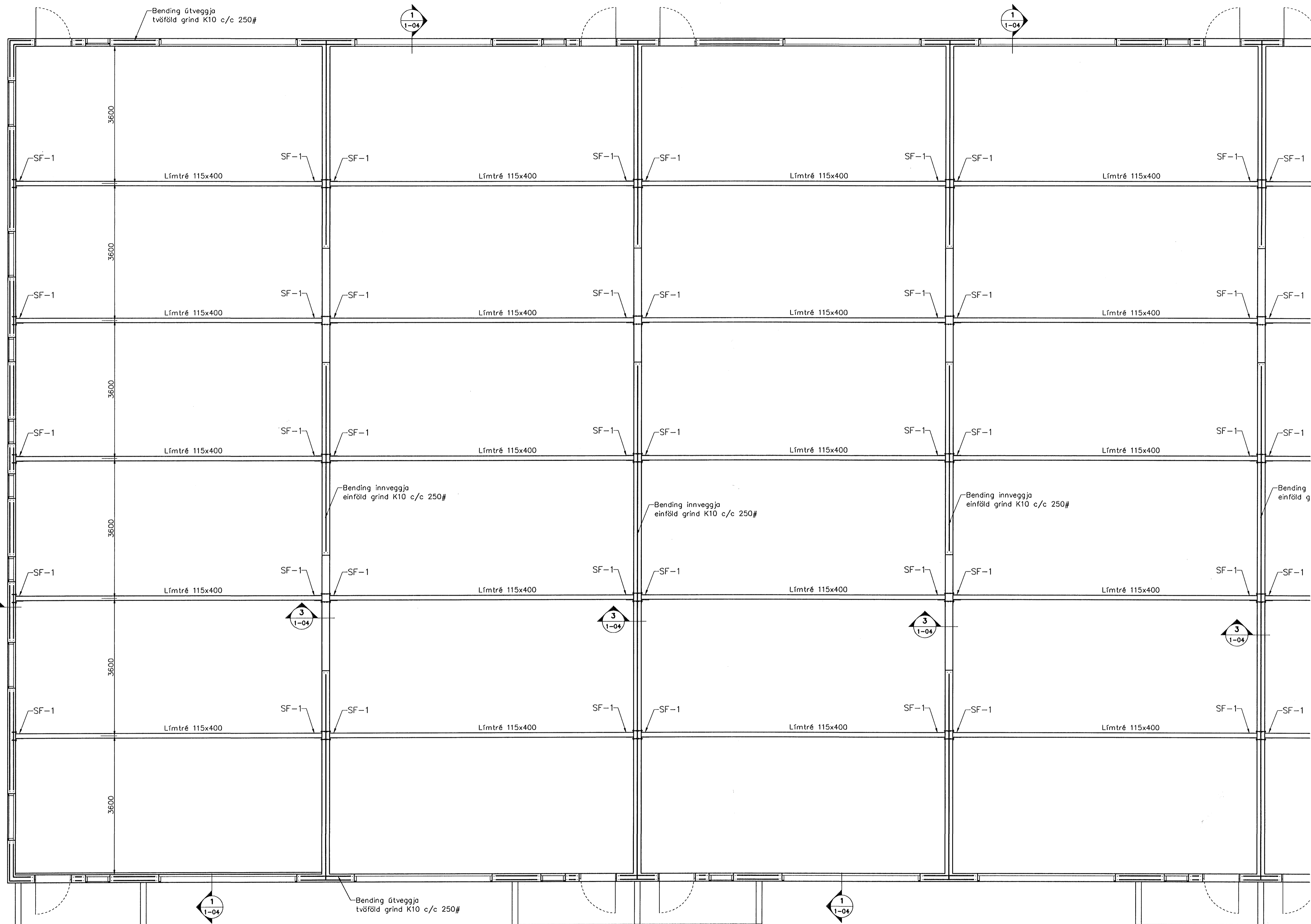
Þakvirki, Grunnmynd, 1:50
