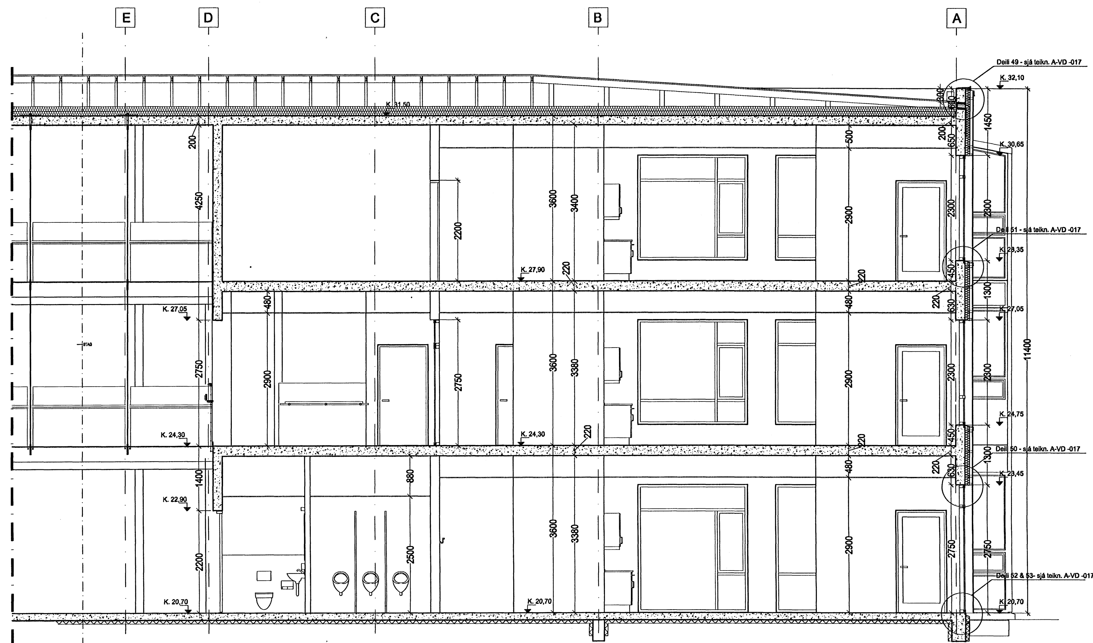
Sneiðing K-K
