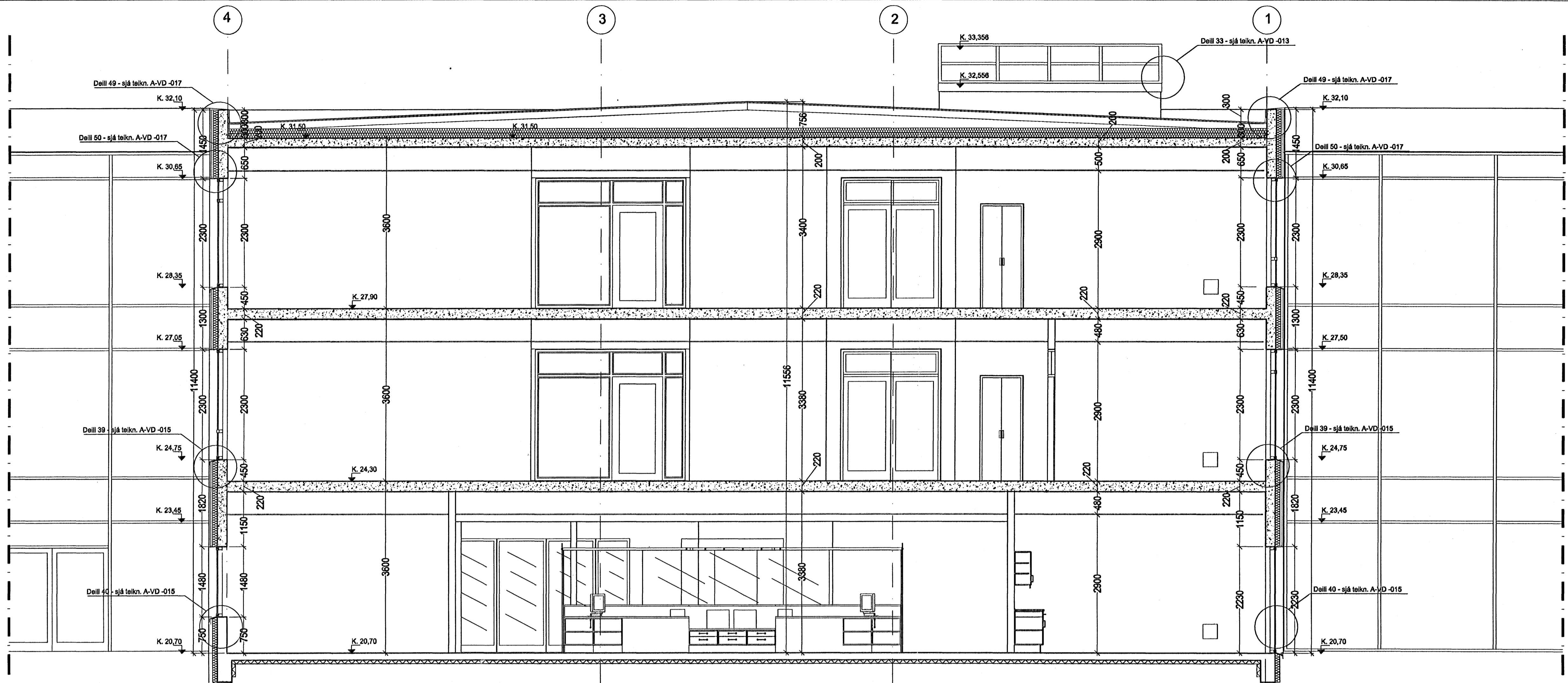
Sneiðing H-H
