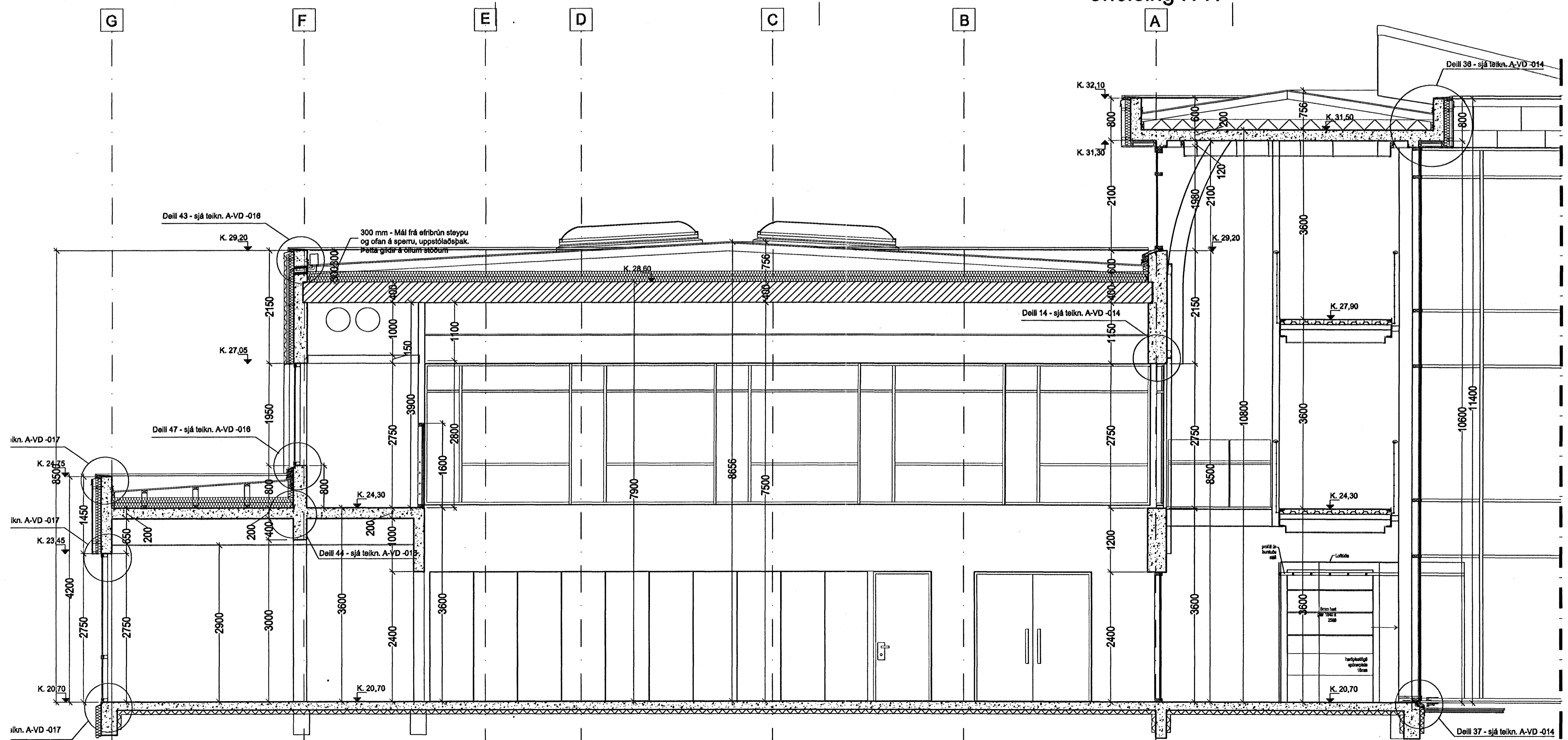
Sneiðing I-I
