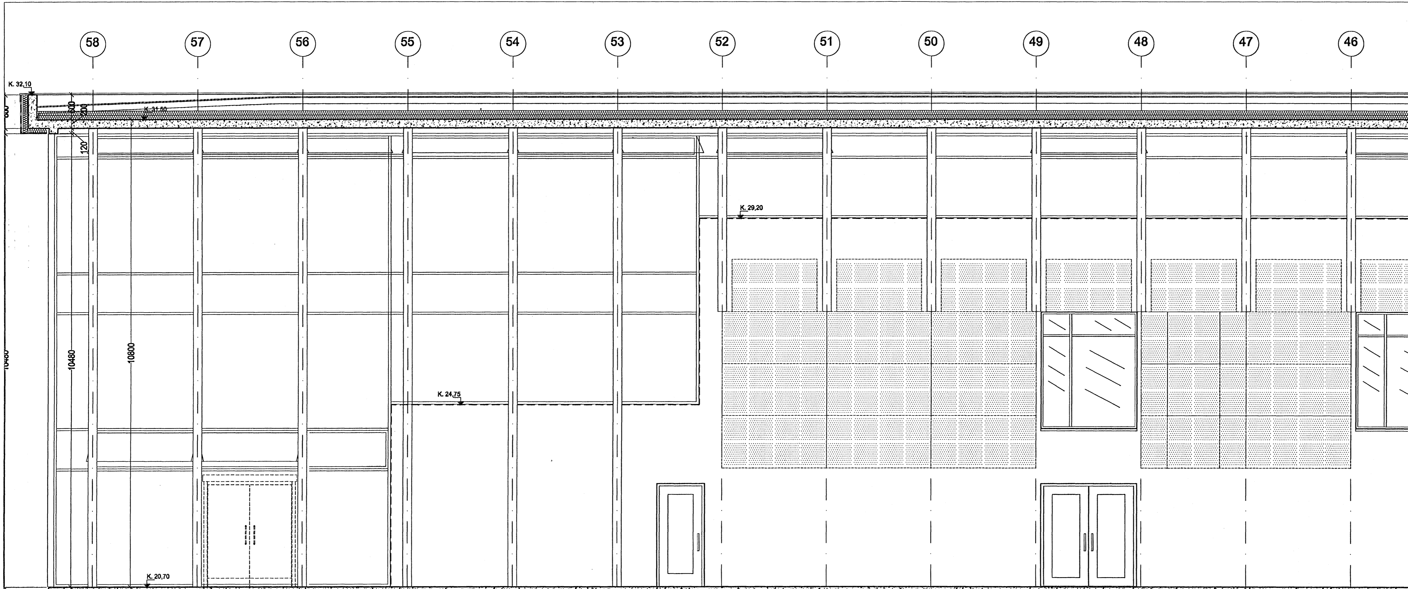
Sneiðing F-F
