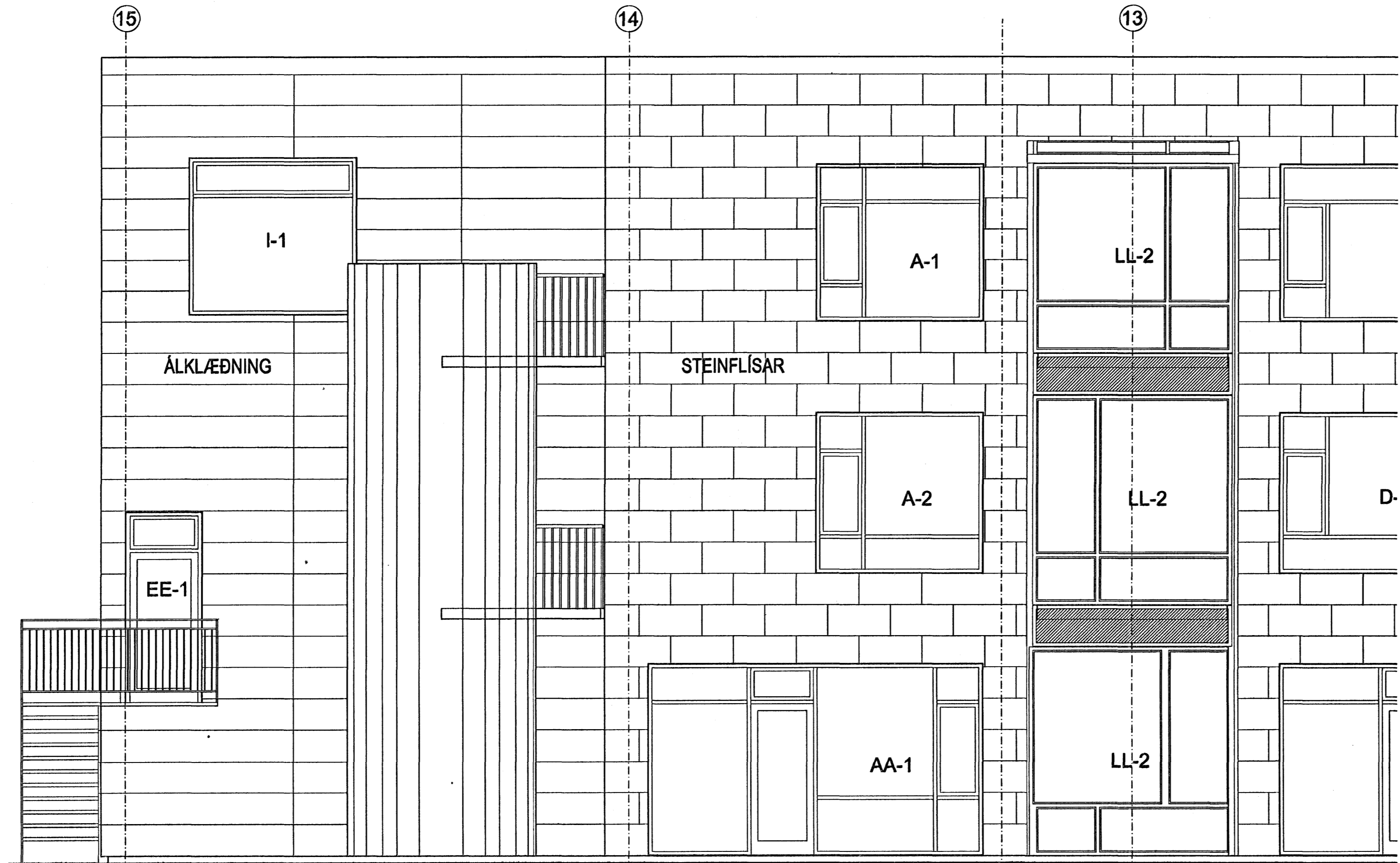
ÚTLIT TIL AUSTURS - BYGGING E
