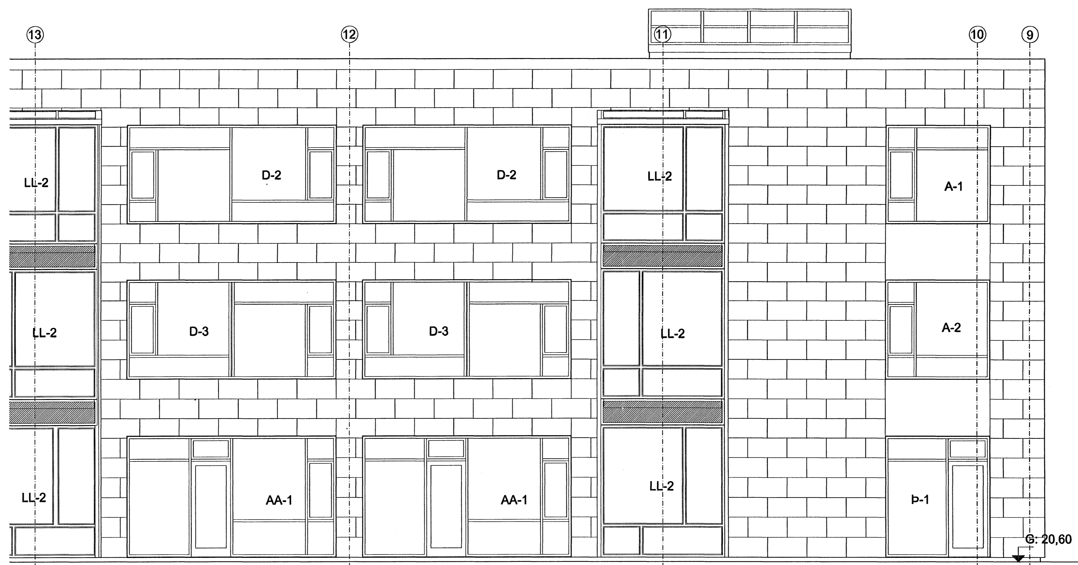
ÚTLIT TIL AUSTURS BYGGING E
