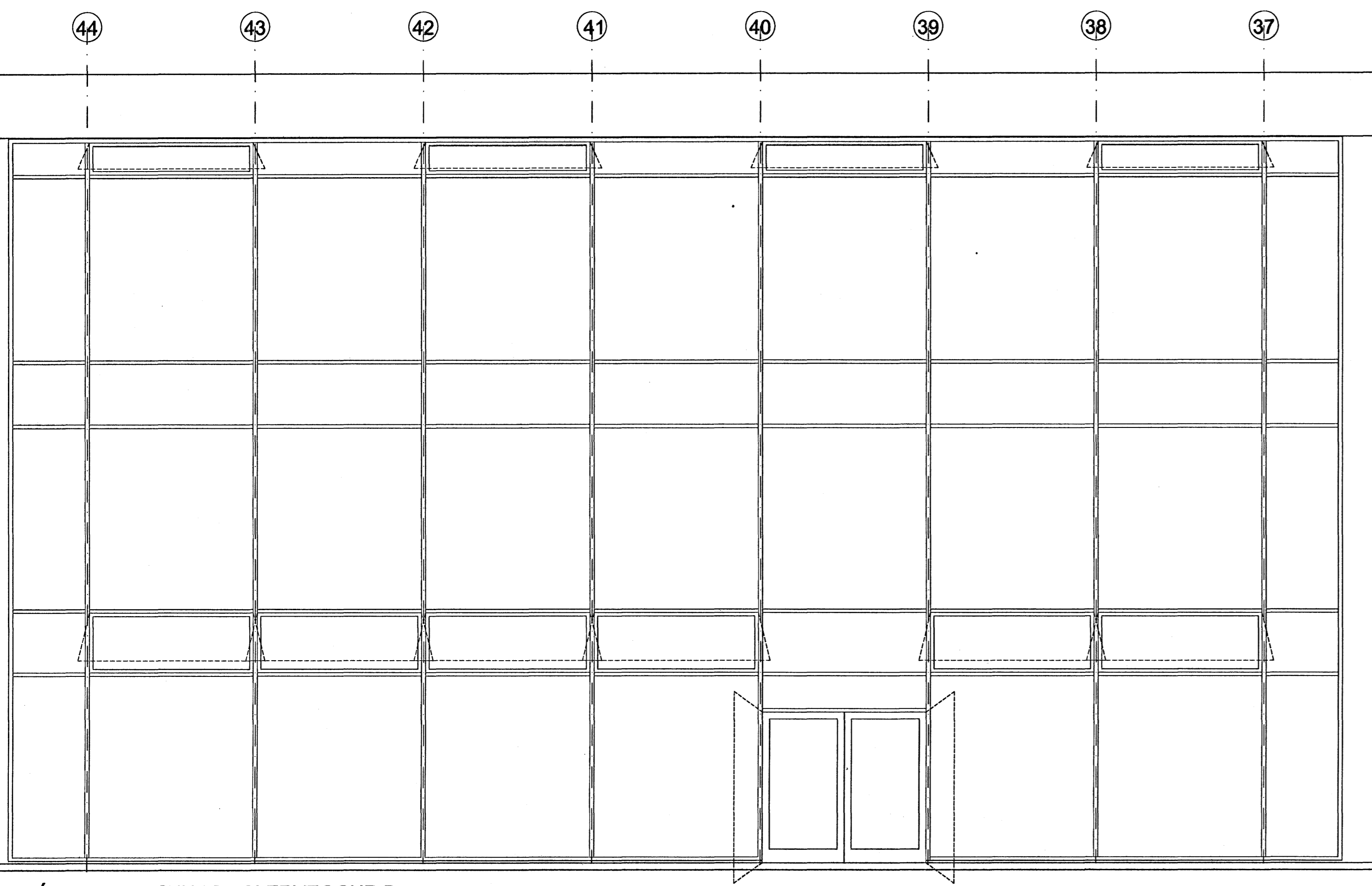
ÚTLIT TIL AUSTURS - GLERVEGGUR B
