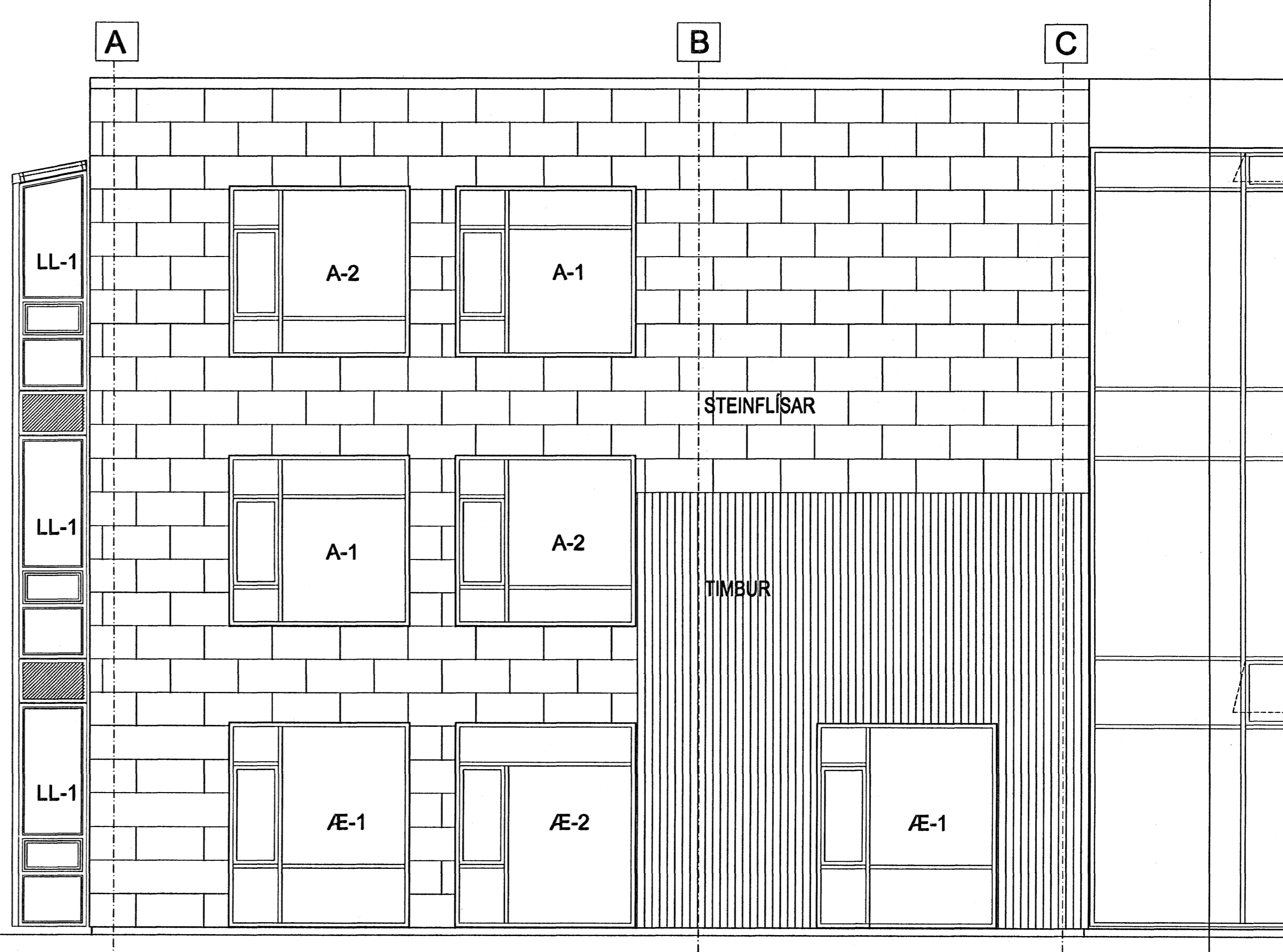
ÚTLIT TIL NORÐURS - BYGGING E
