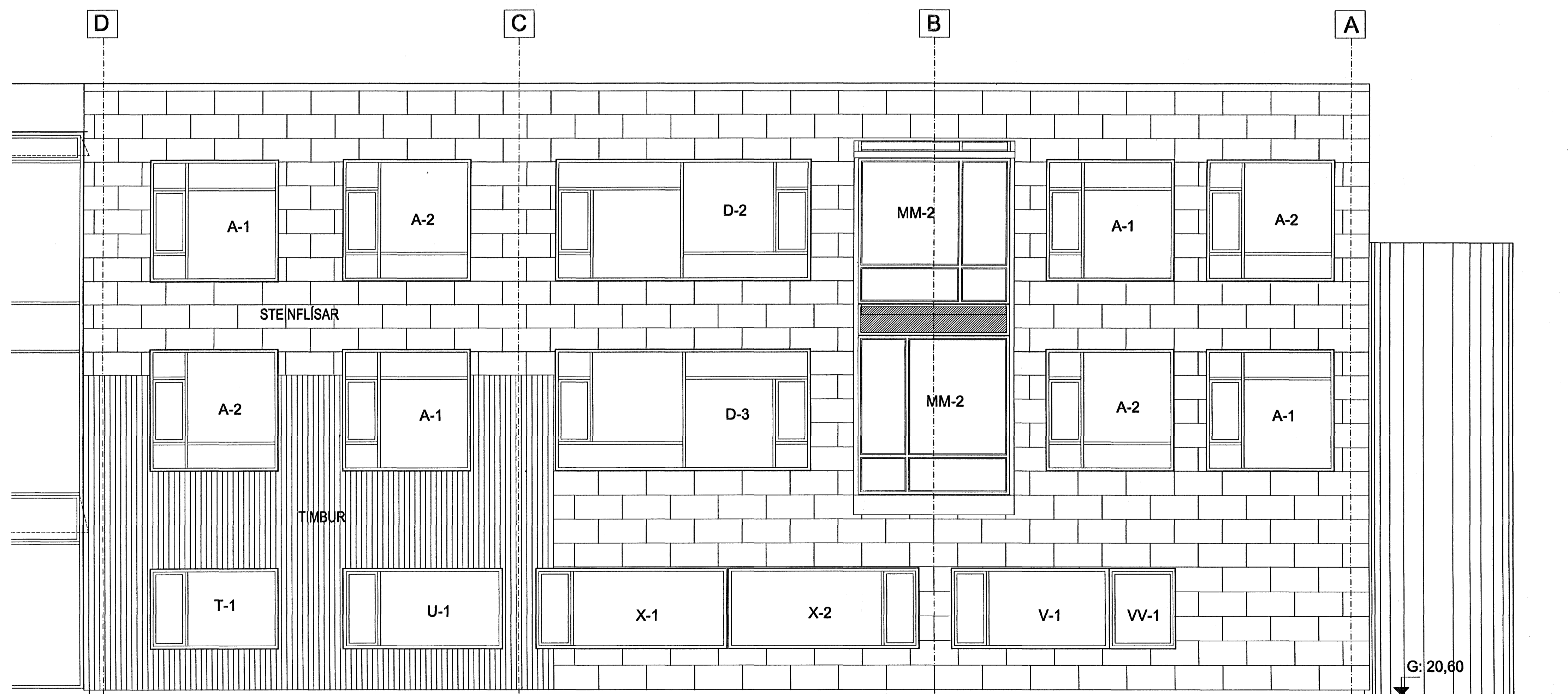
ÚTLIT TIL SUÐURS - BYGGING C
