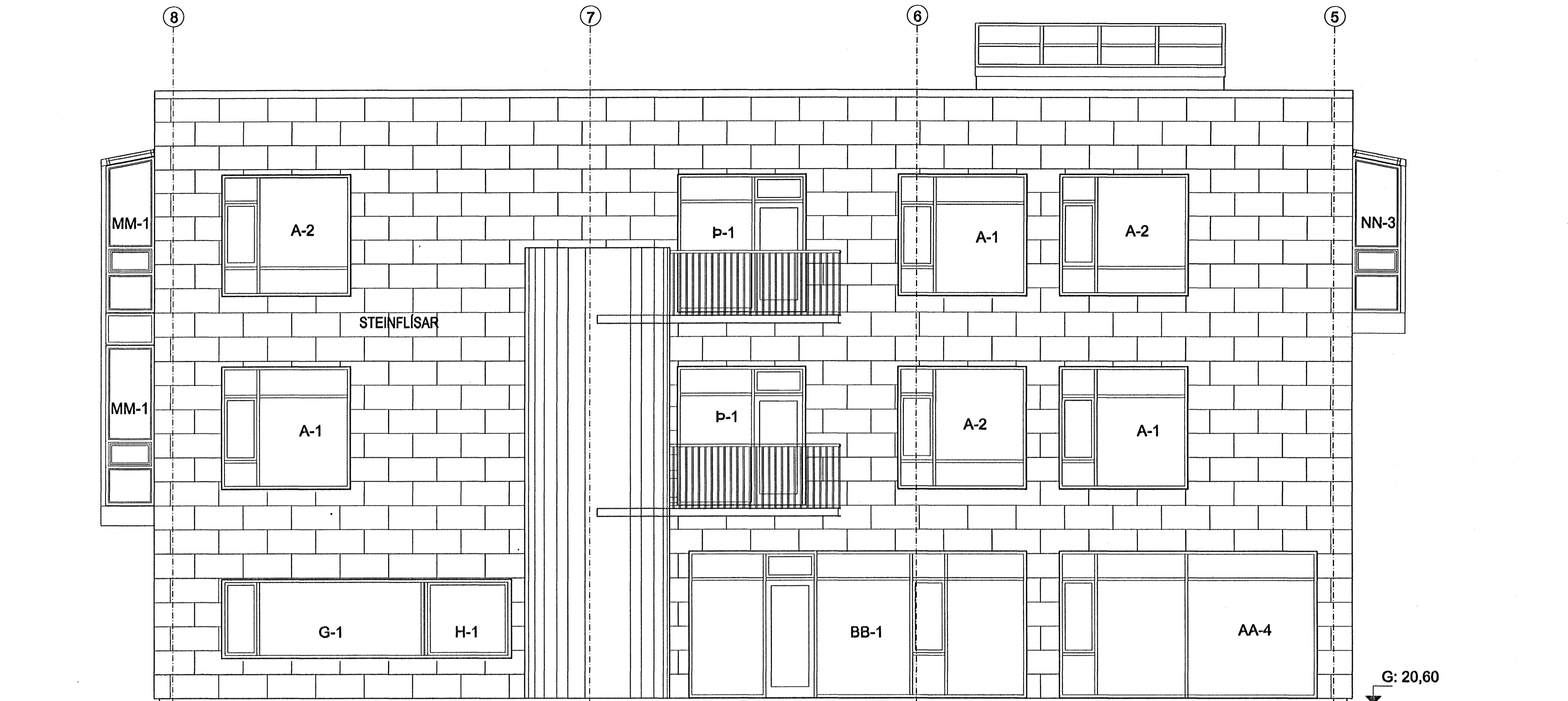
ÚTLIT TIL AUSTURS - BYGGING C
