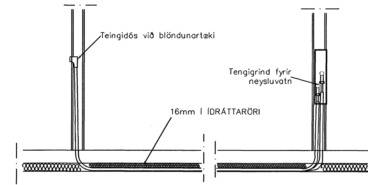
TENGING NEYSLUVATNSLAGNA 1:20
