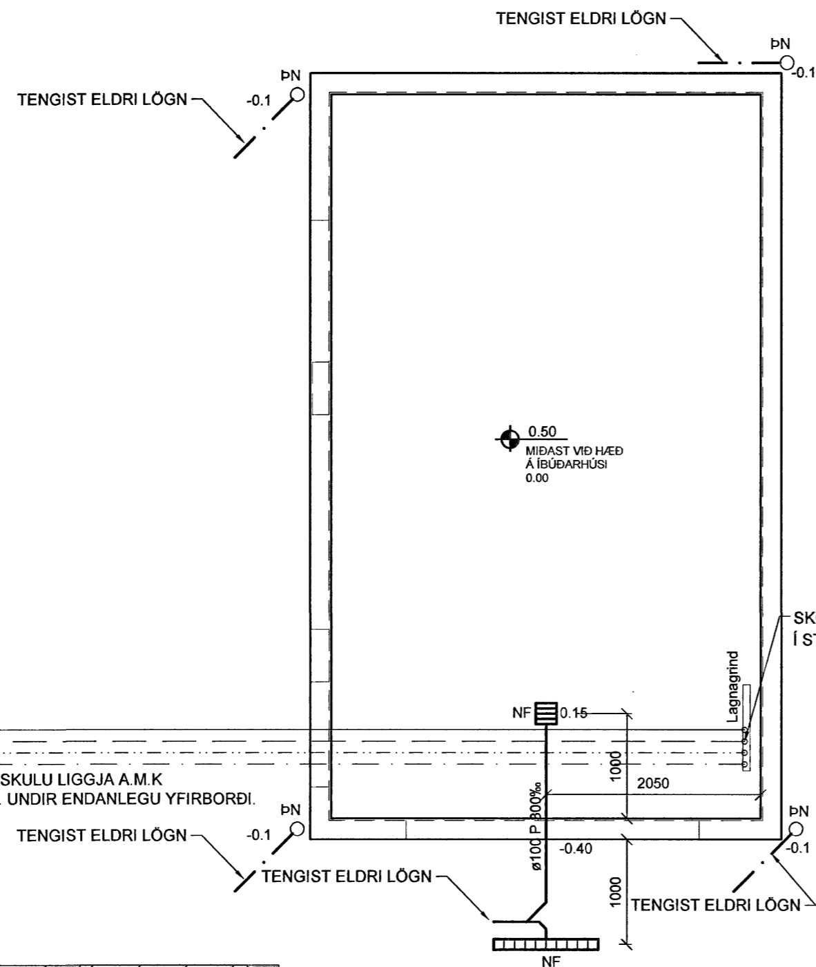
GRUNNMYND LAGNA Í JÖRÐ 1:50
