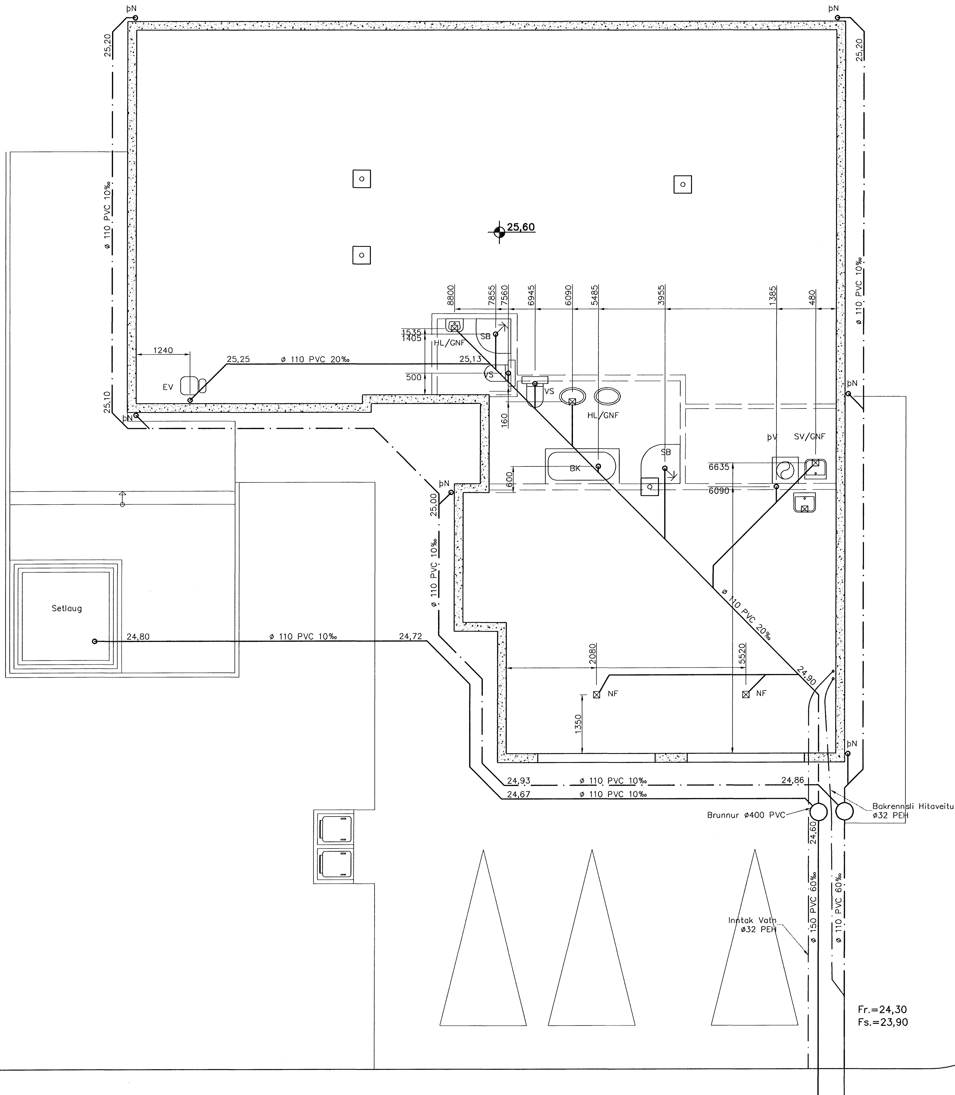
Grunnlagnir, Grunnmynd, 1:50
