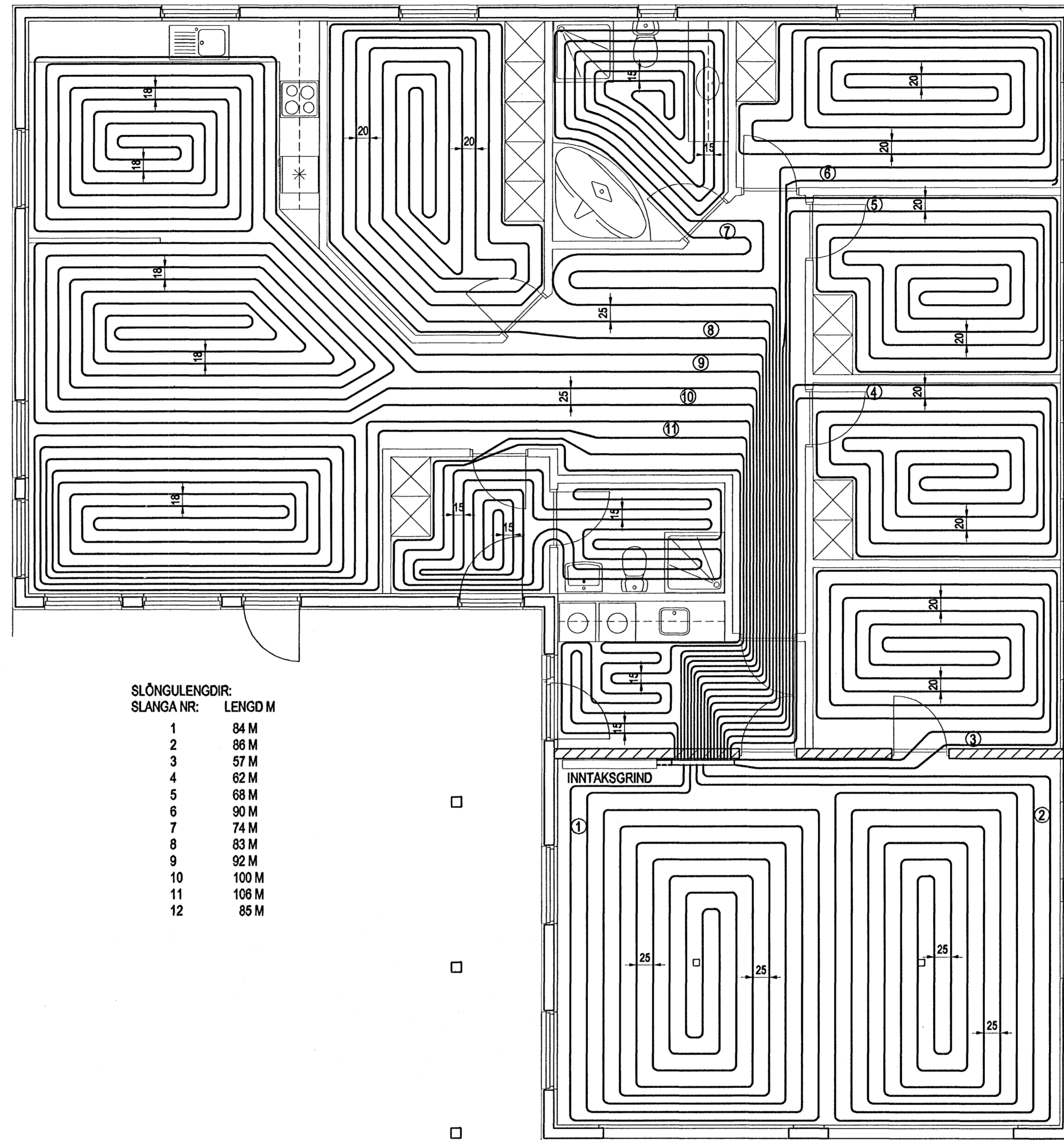
GÓLFHITALAGNIR - GRUNNMYND MKV. 1:50
