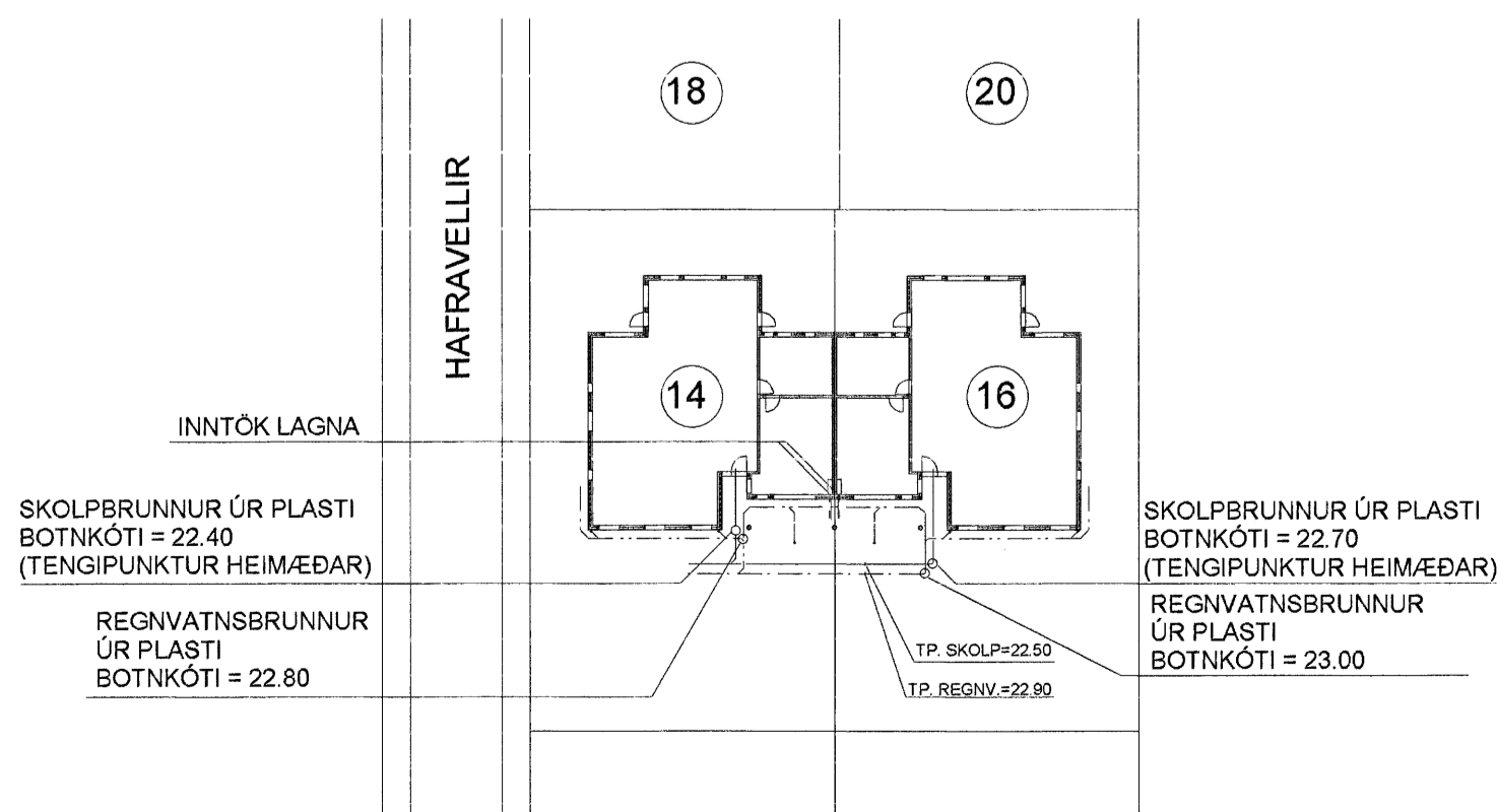
AFSTÖÐUMYND MKV. 1:500
