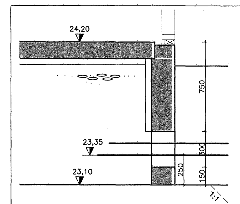
KÓTAR, SKÝRINGAR Mkv. 1:20
