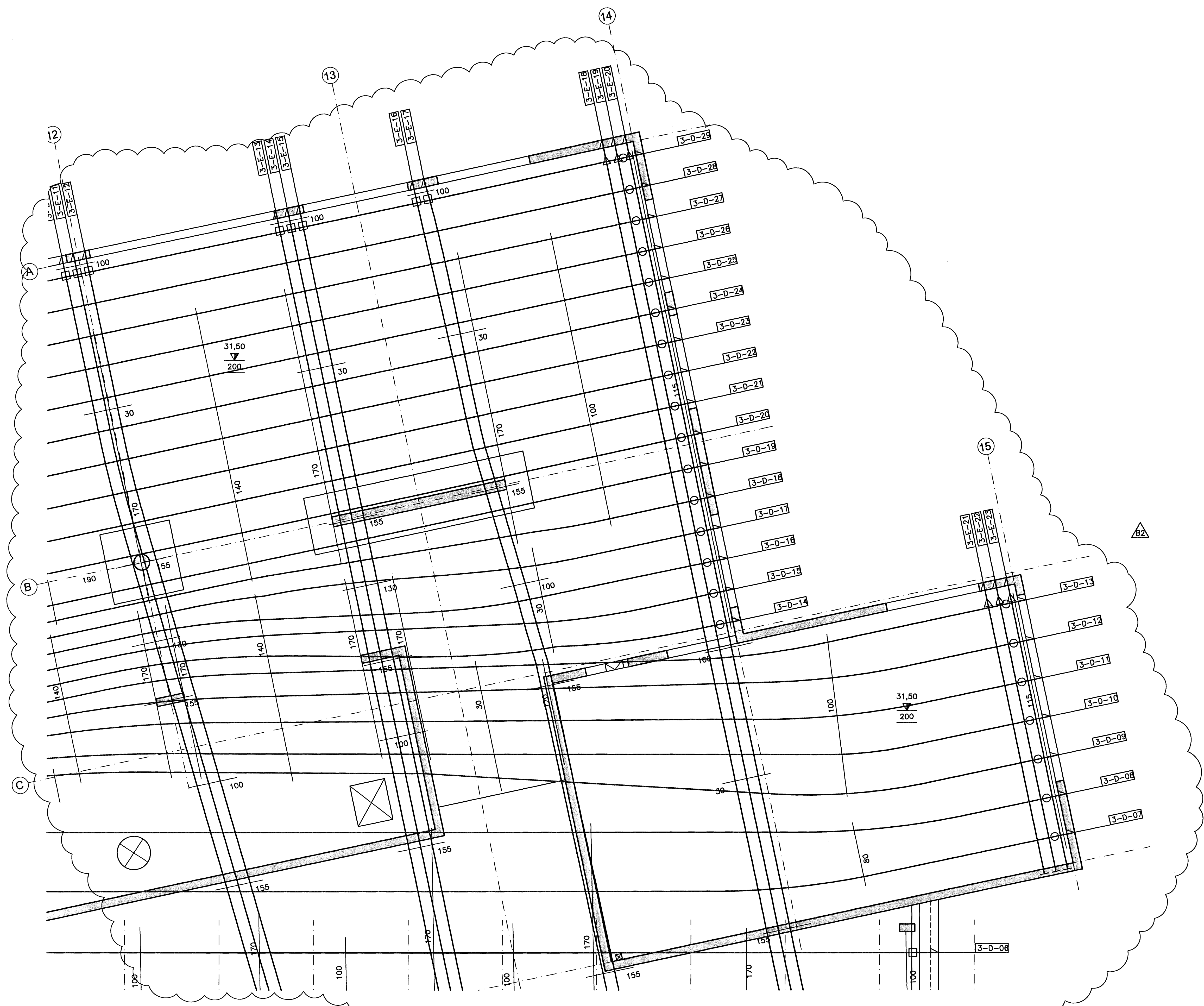
3. HÆÐ. GRUNNMYND. EFTIRSPENNUKAPLAR MKV. 1
