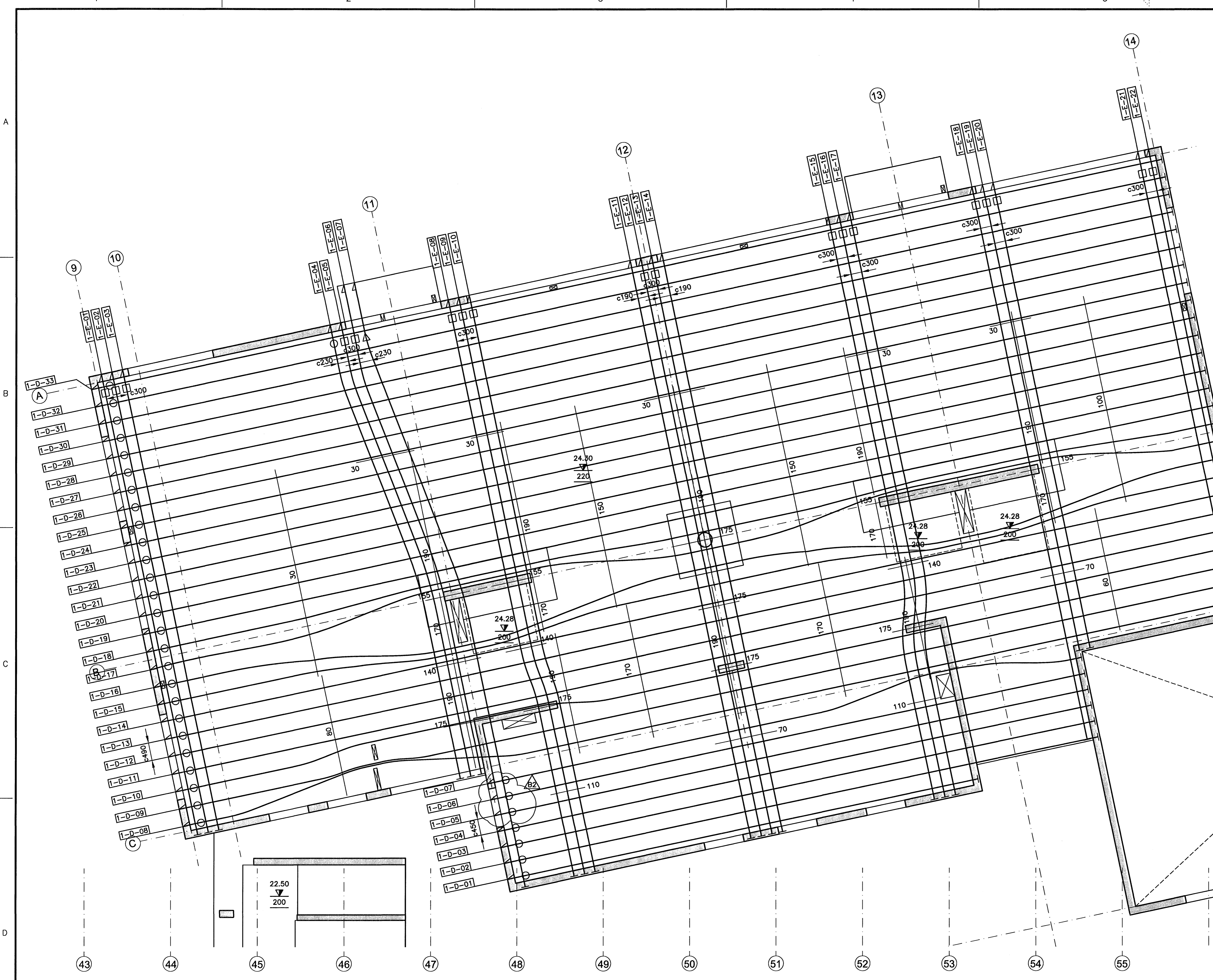
1. HÆÐ, GRUNNMYND, EFTIRSPENNUKAPLAR MKV. 1
