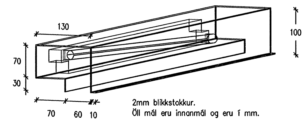
Ljósastokkur 1:5
