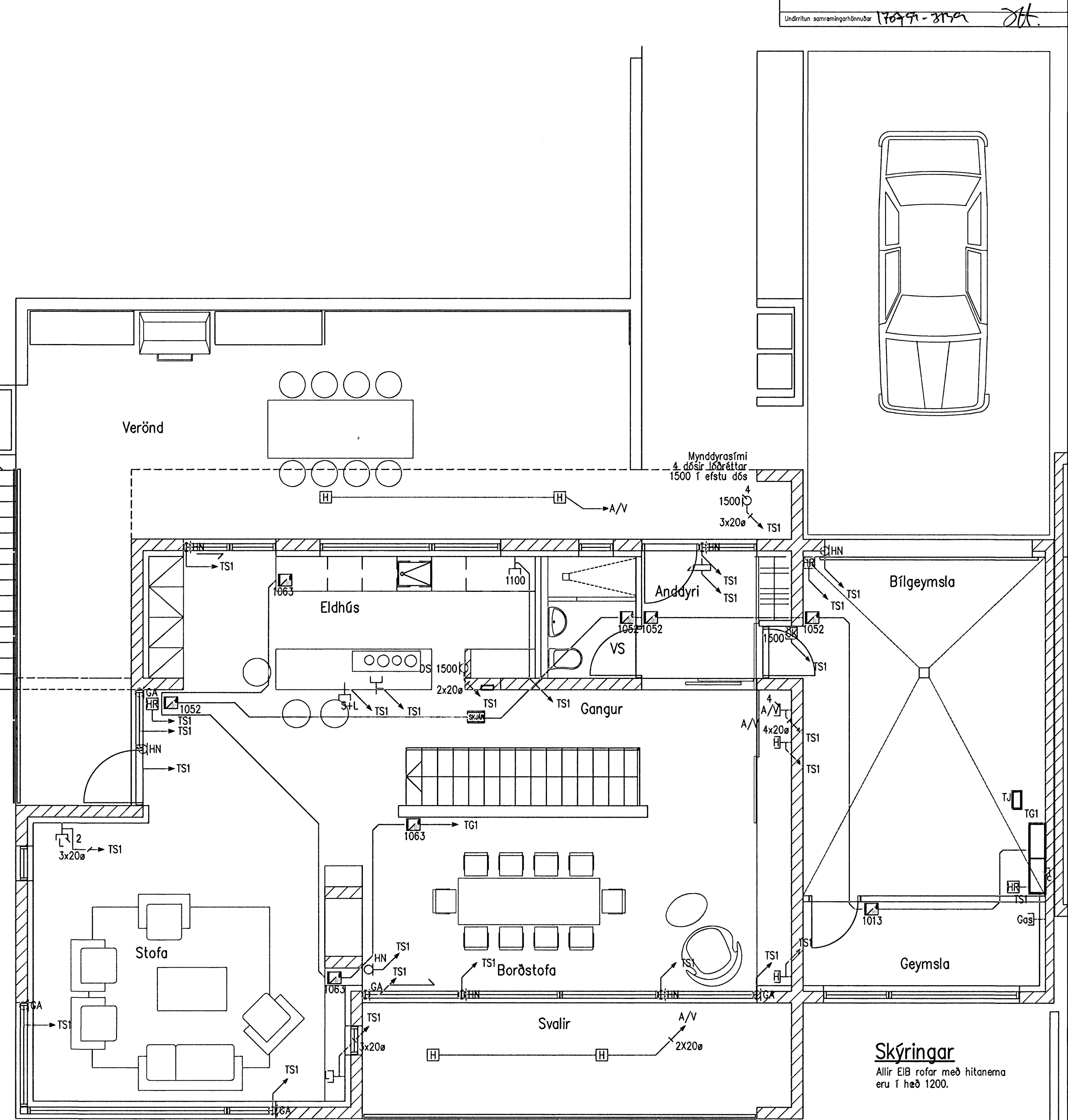
Grunnmynd 2.hæð, smáspenna, 1:50
