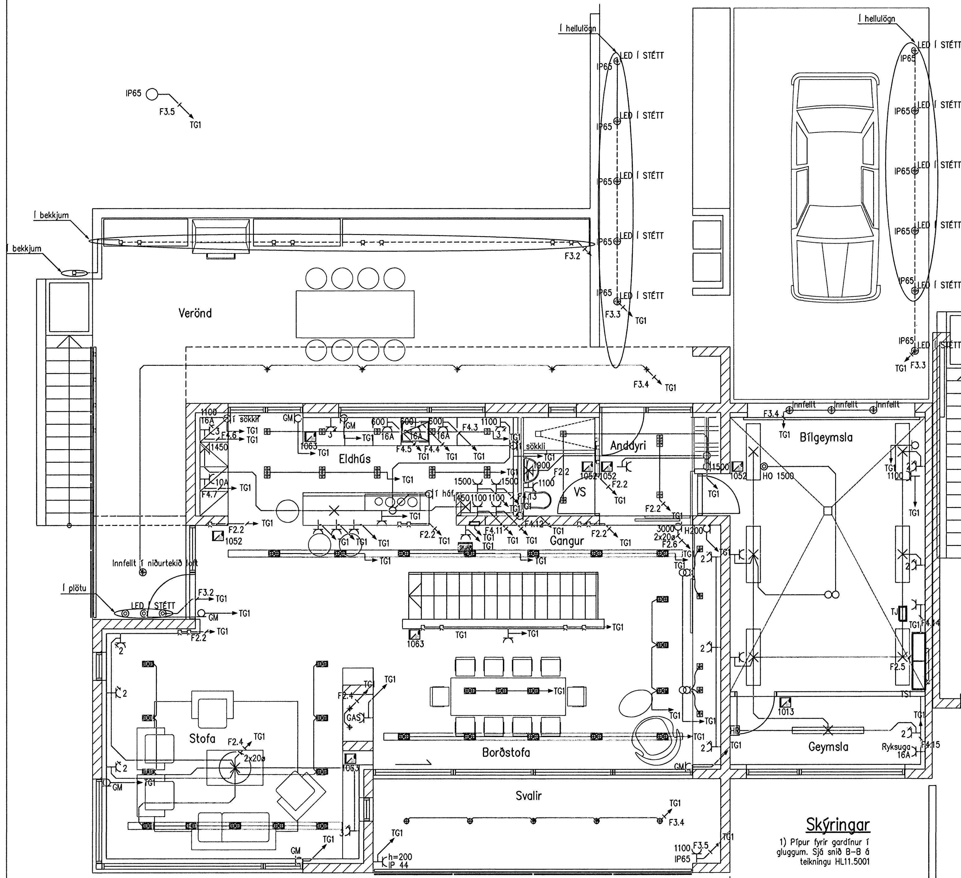
Grunnmynd 2.hæð, lágspenna, 1:50
