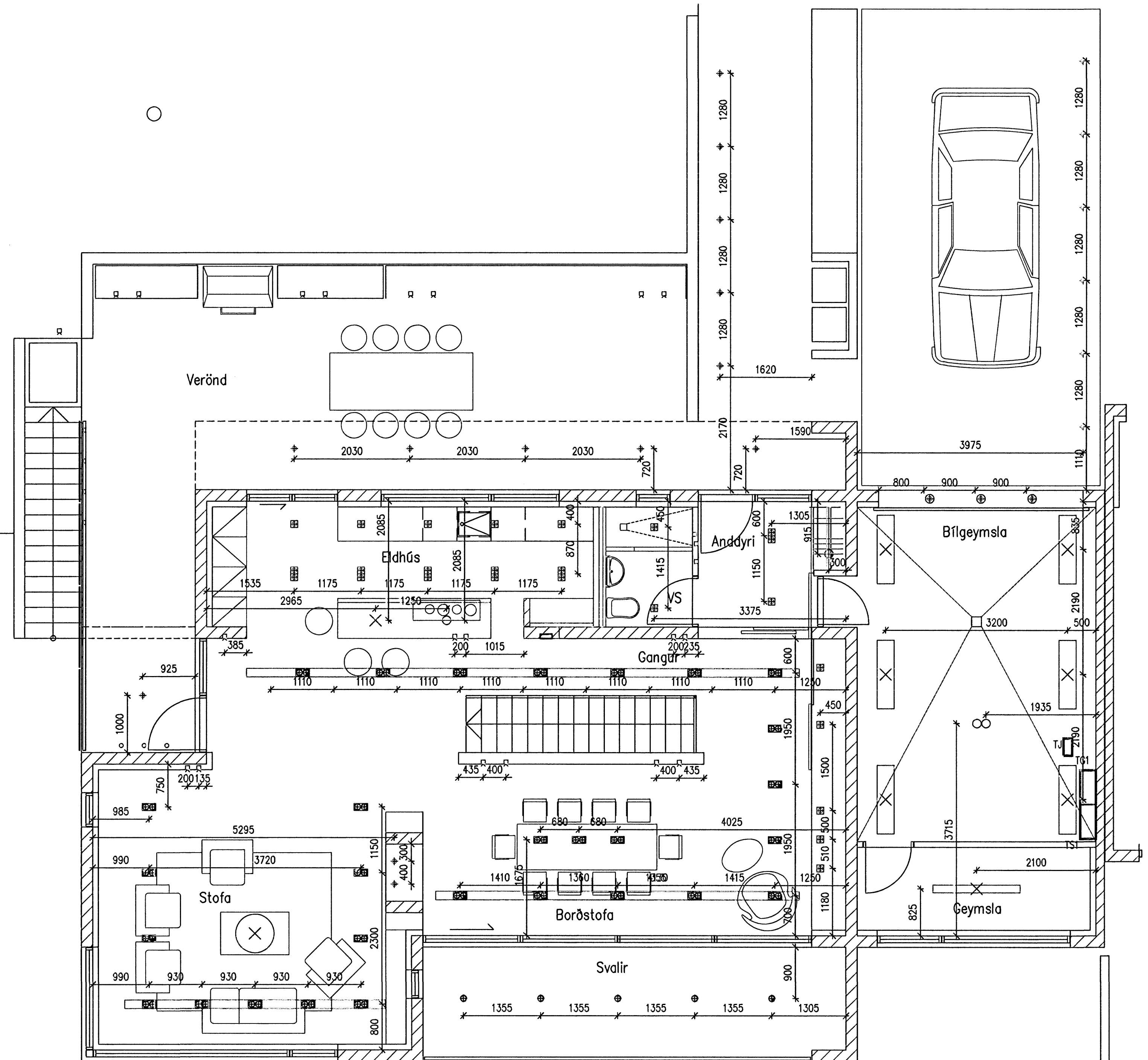
Grunnmynd 2.hæð, 1:50
