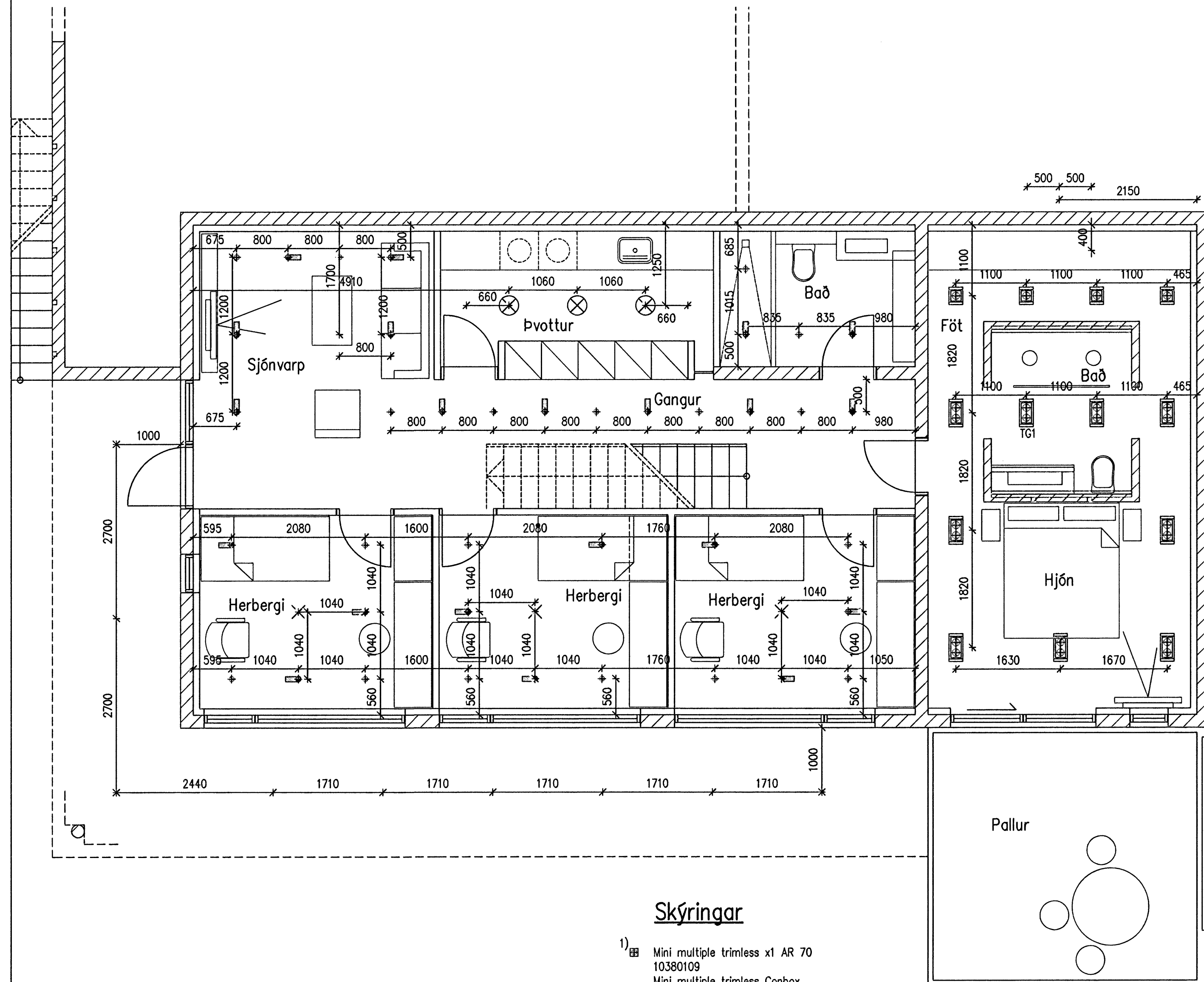
Grunnmynd 1.hæð, 1:50
