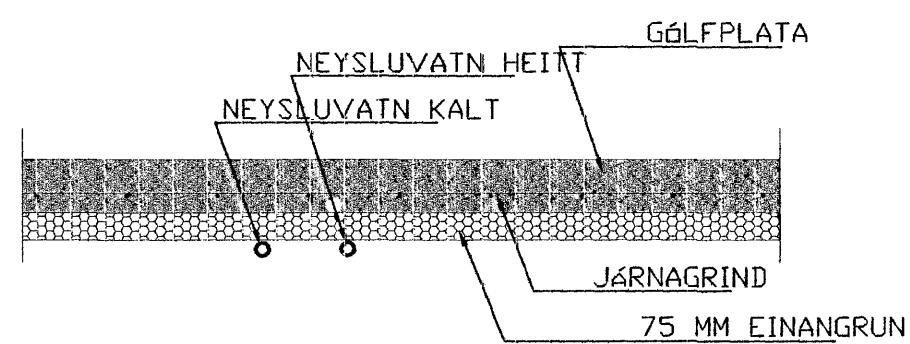
SNID Í NEYSLUVATN Í GÖLFI 1:20 RÖR Í RÖR
