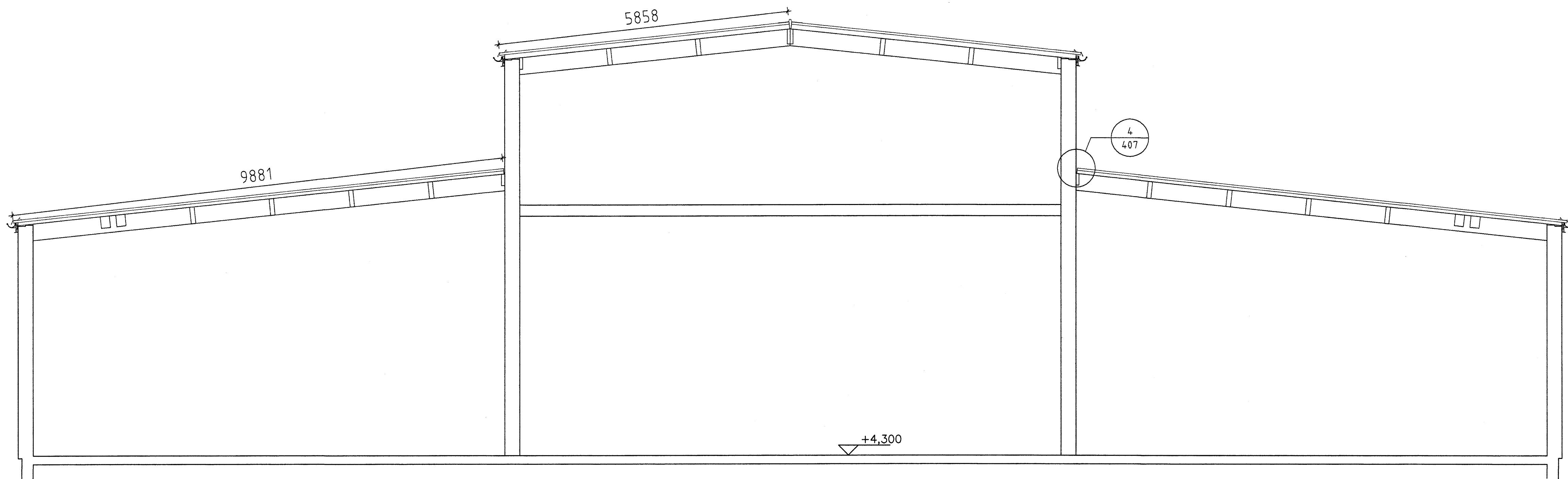
Dversnið B Mkv. 1:50 401
