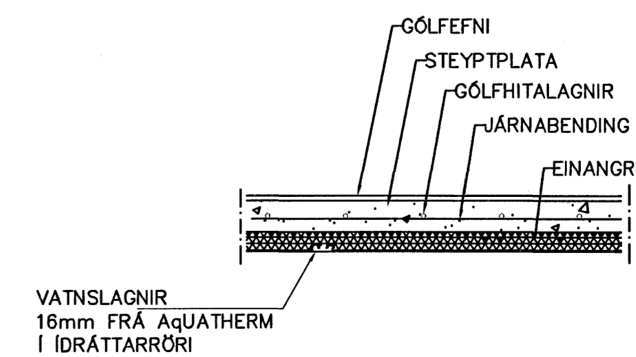
LAGNIR, SNIÐ, 1:20
