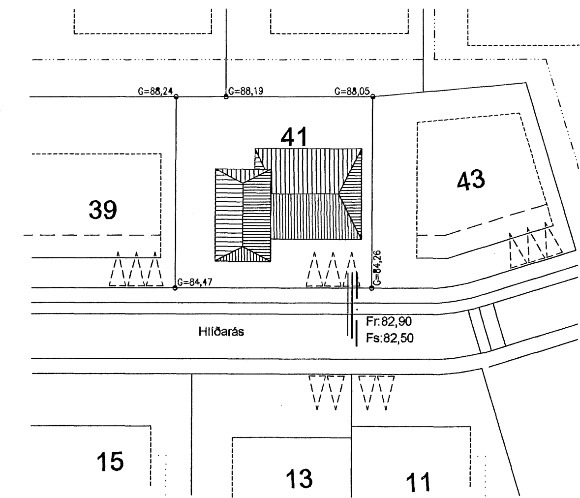
Afstöðumynd 1:500
