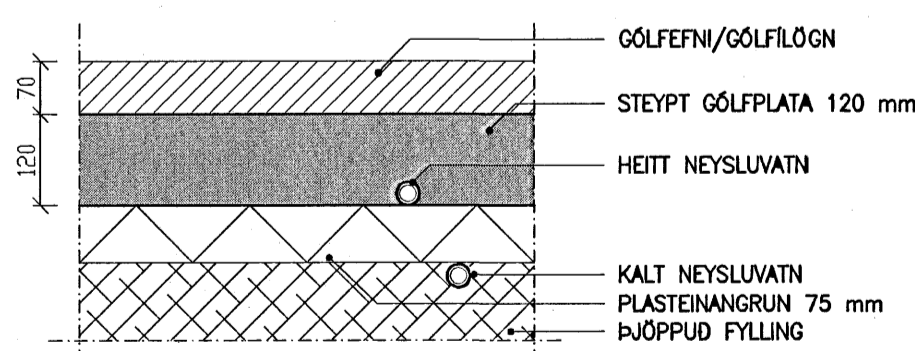
FRÁGANGUR LAGNA Í GÓLFPLÖTU
