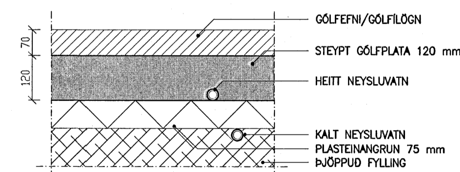
FRÁGANGUR LAGNA Í GÓLFPLÖTU
