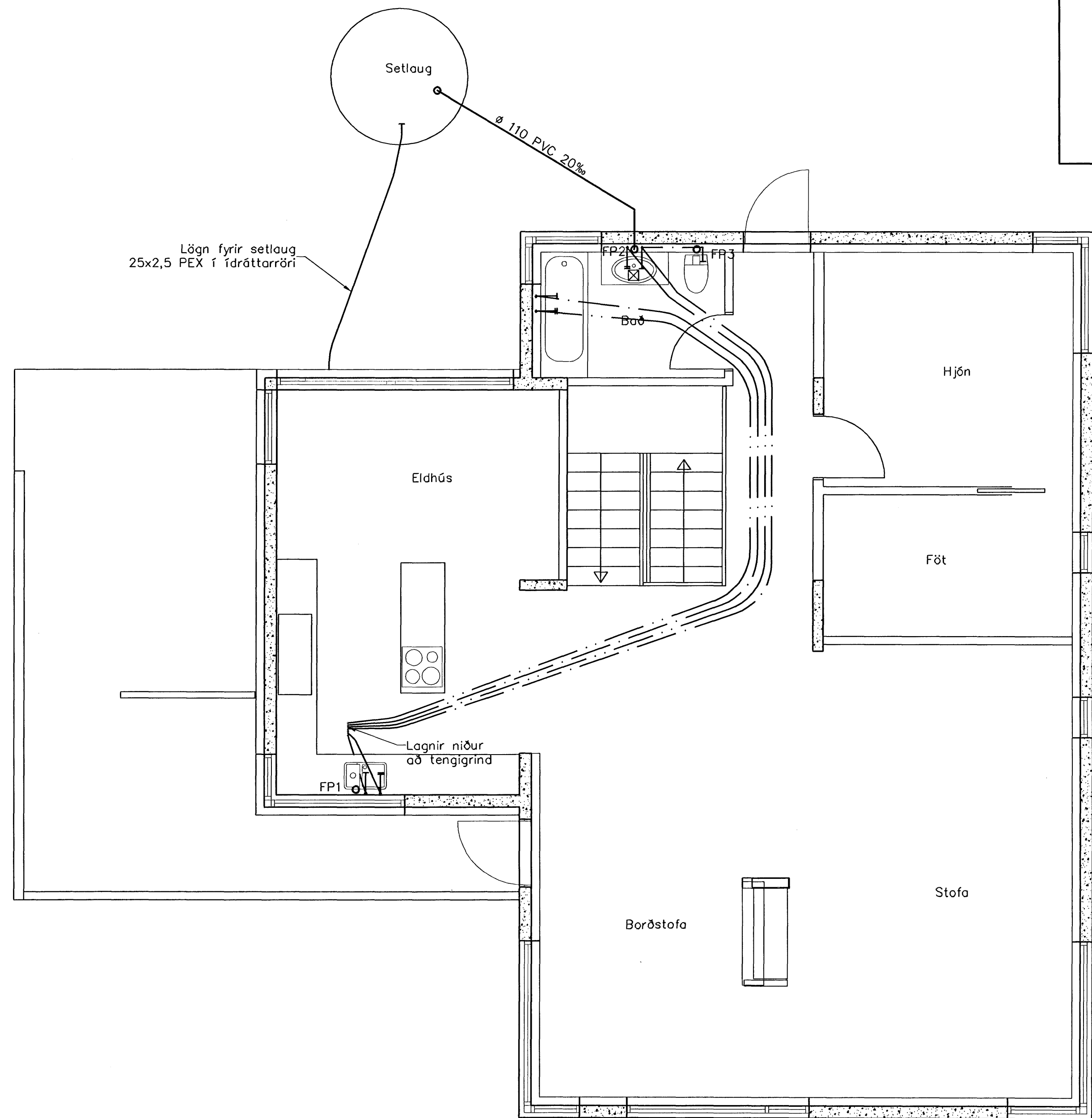
Neysluvatnslagnir 2. hæð, 1:50
