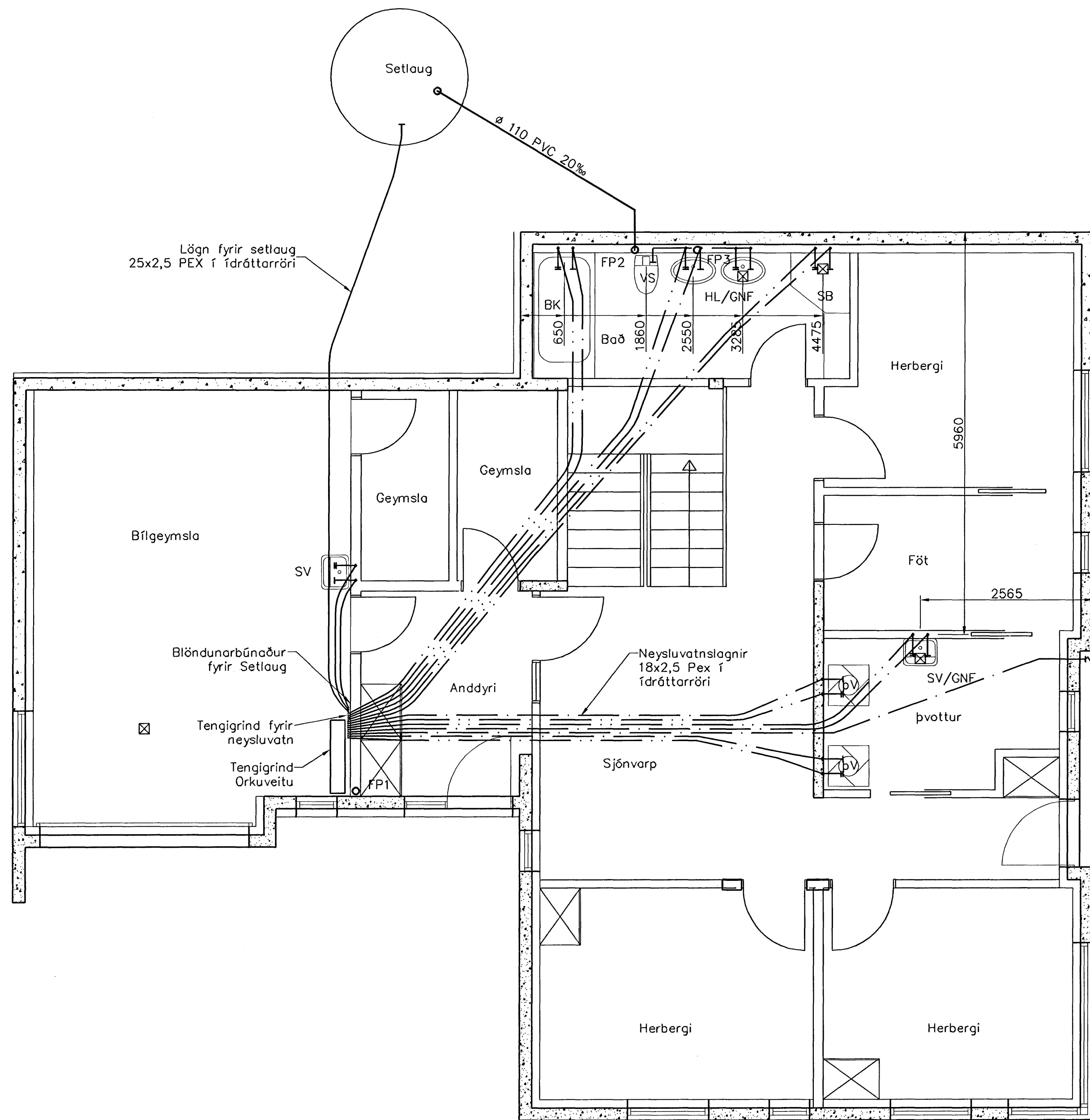
Neysluvatnslagnir 1. hæð, 1:50
