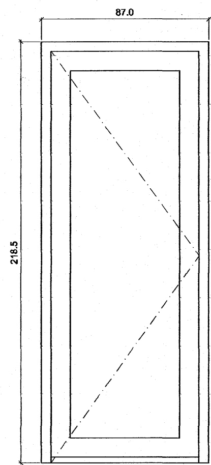
H3 2stk. úthúrdir- vinstri hengdar Opnast út
