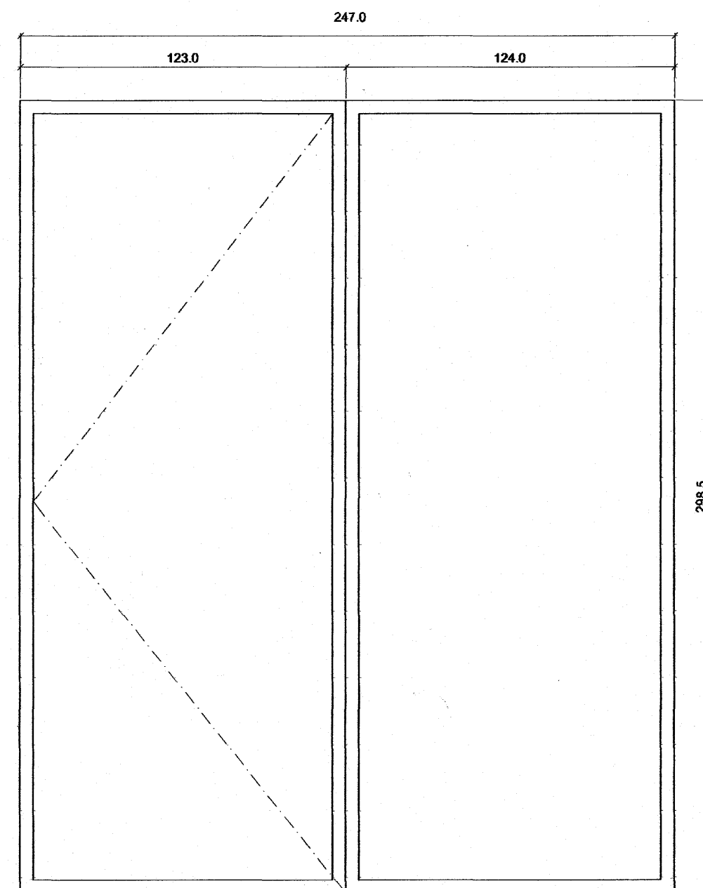
RH2 1.stk. Rennihuró.
