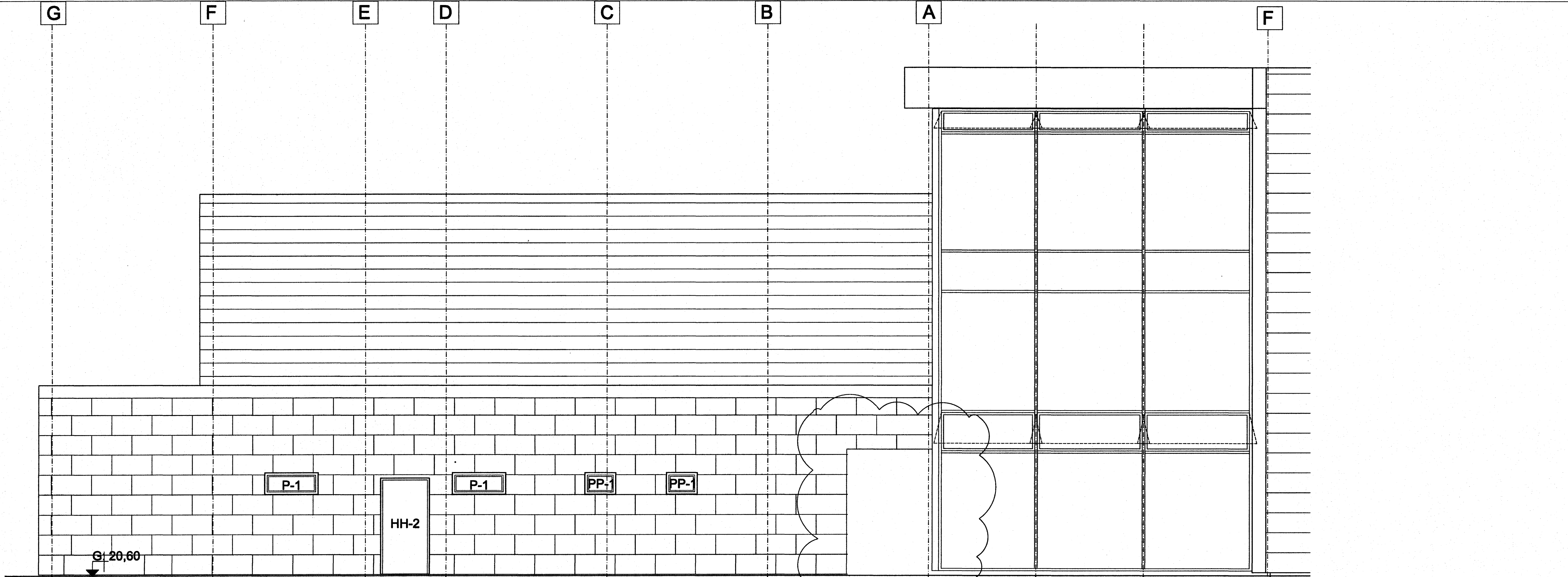
ÚTLIT TIL SUÐURS - BYGGING F
