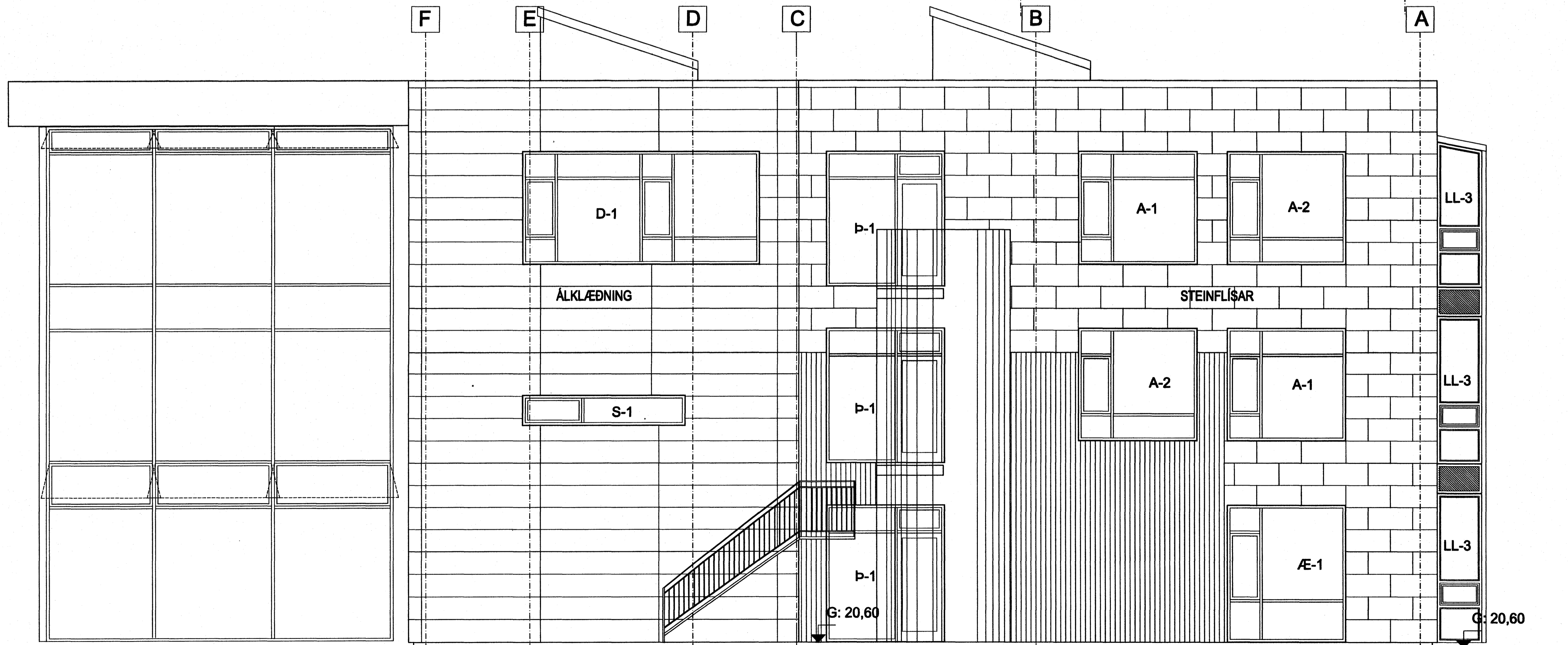
ÚTLIT TIL SUÐURS - BYGGING E
