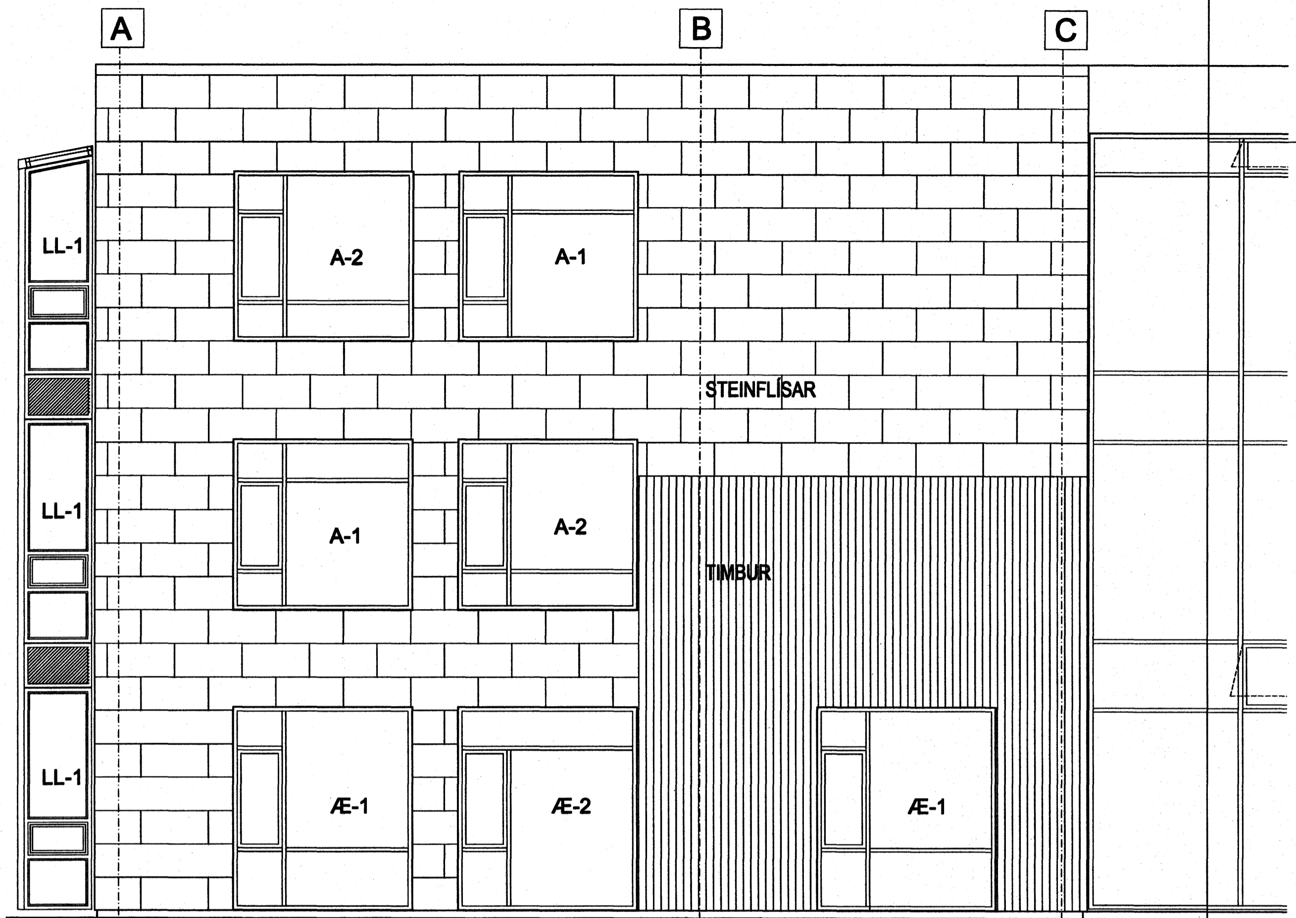
ÚTLIT TIL NORÐURS - BYGGING E
