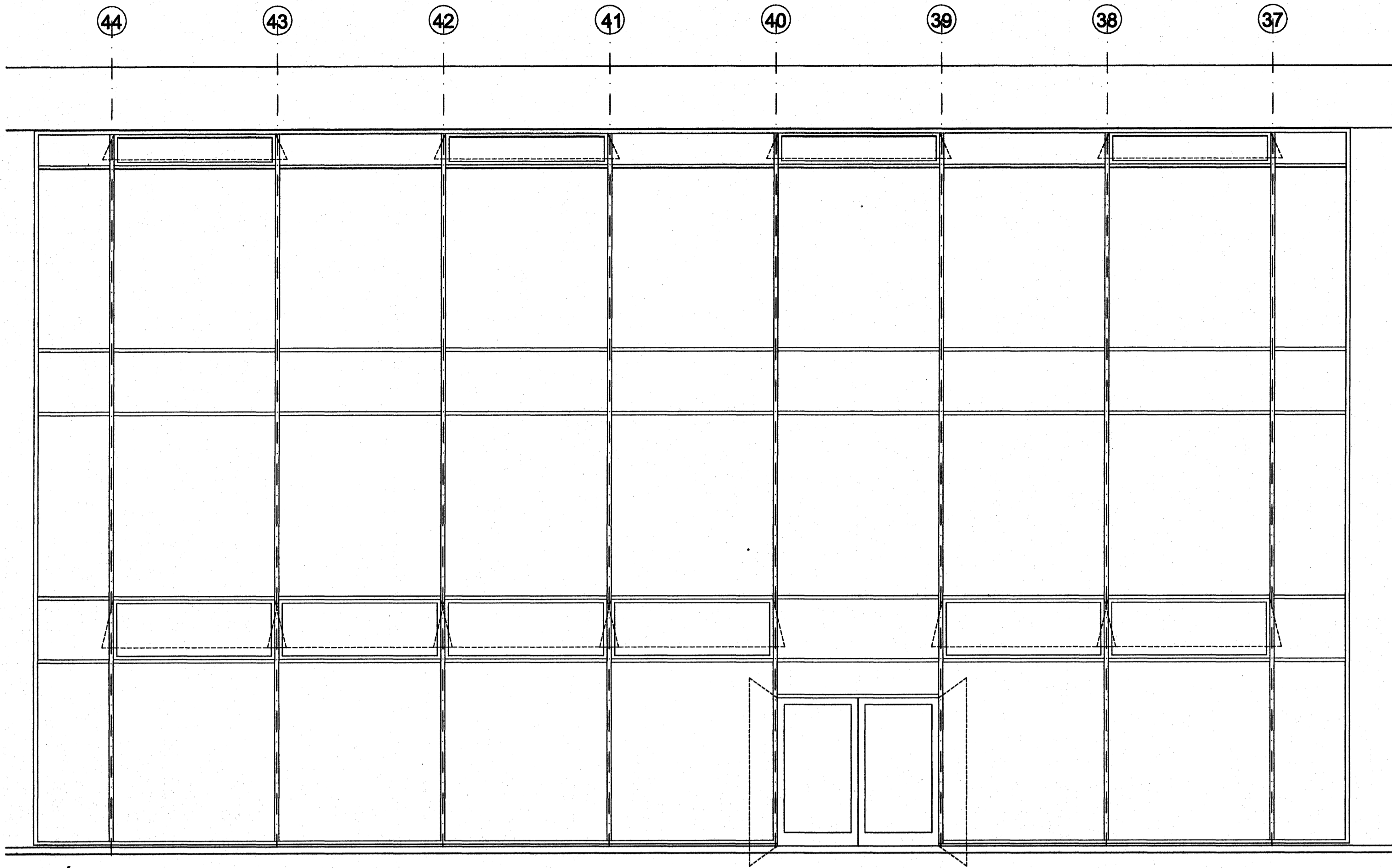
ÚTLIT TIL AUSTURS - GLERVEGGUR B
