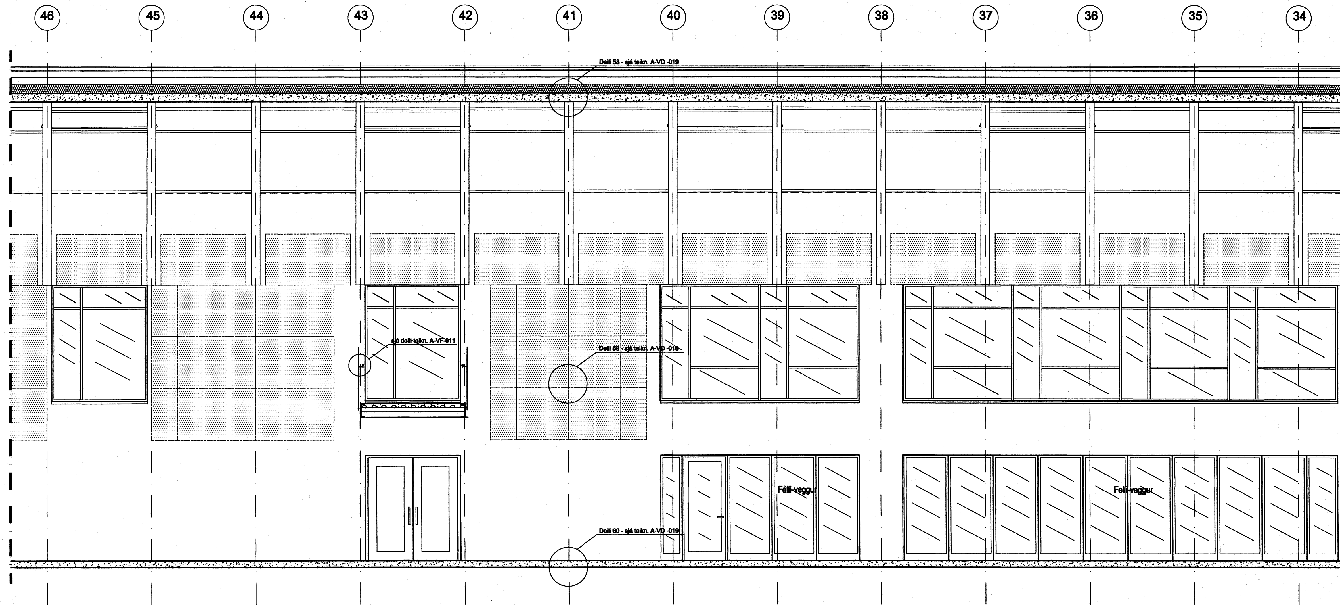
Sneiðing F-F
