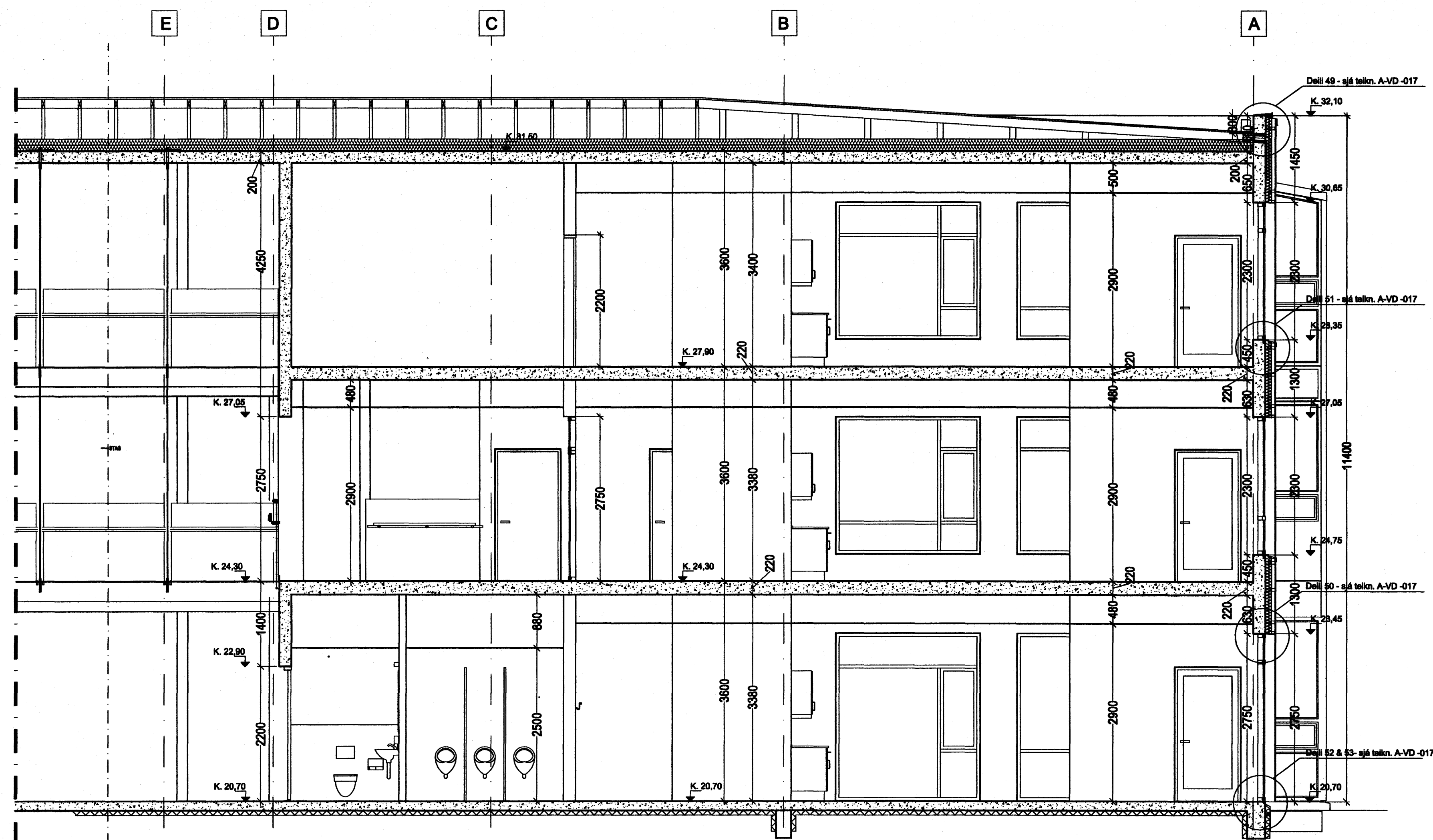
Sneiðing K-K
