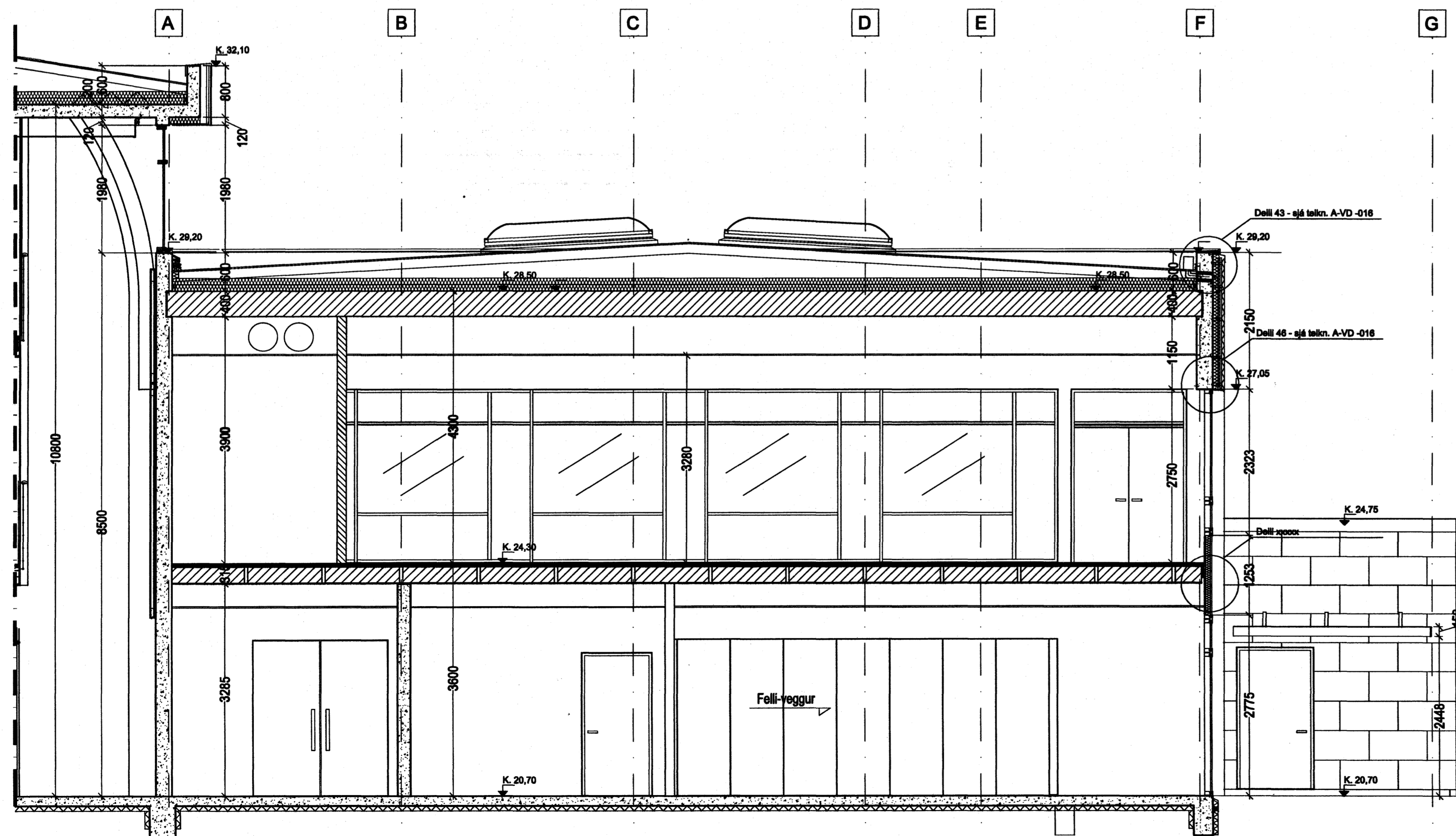
Sneiðing M-M
