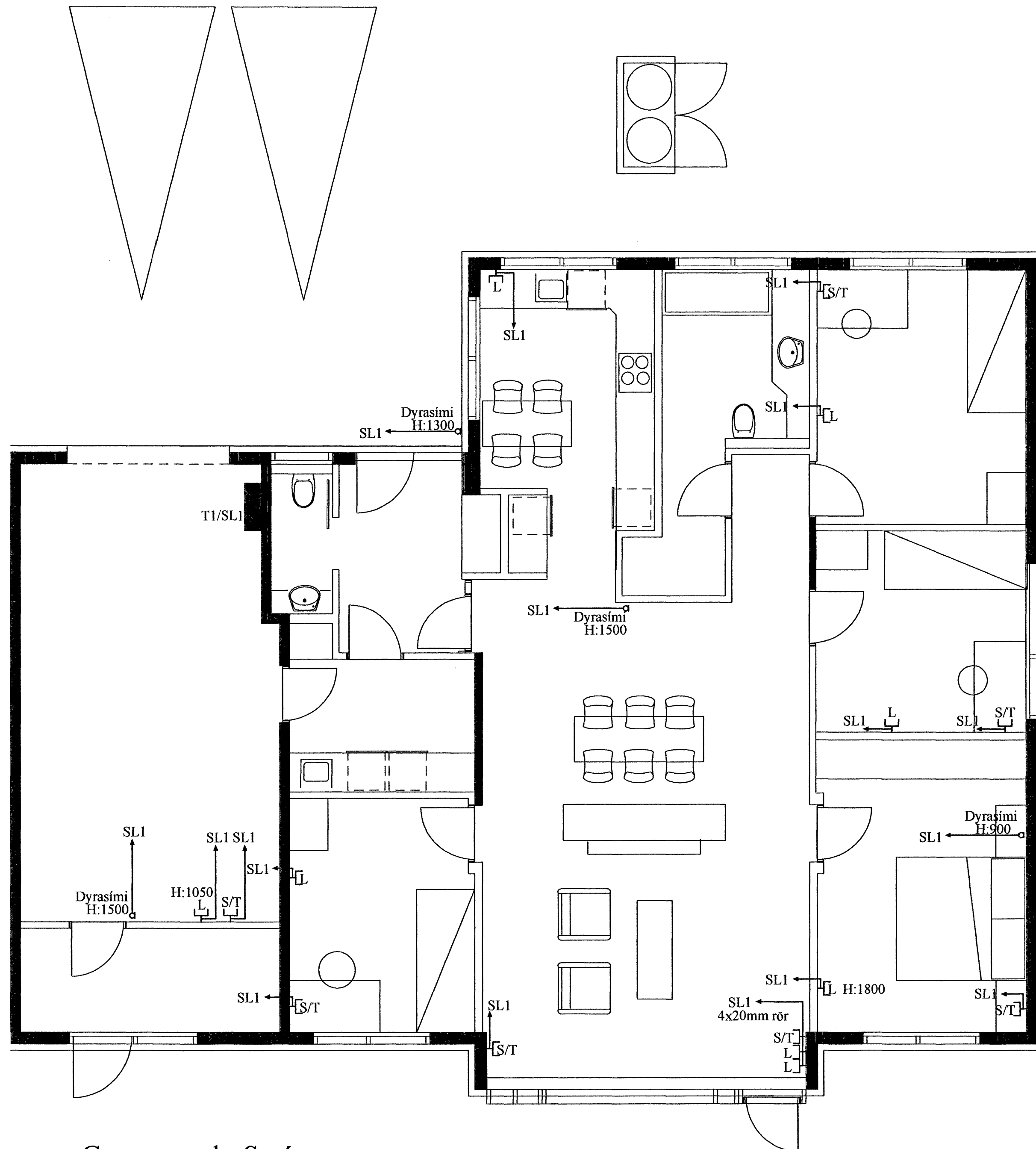
Grunnmynd - Smáspenna
