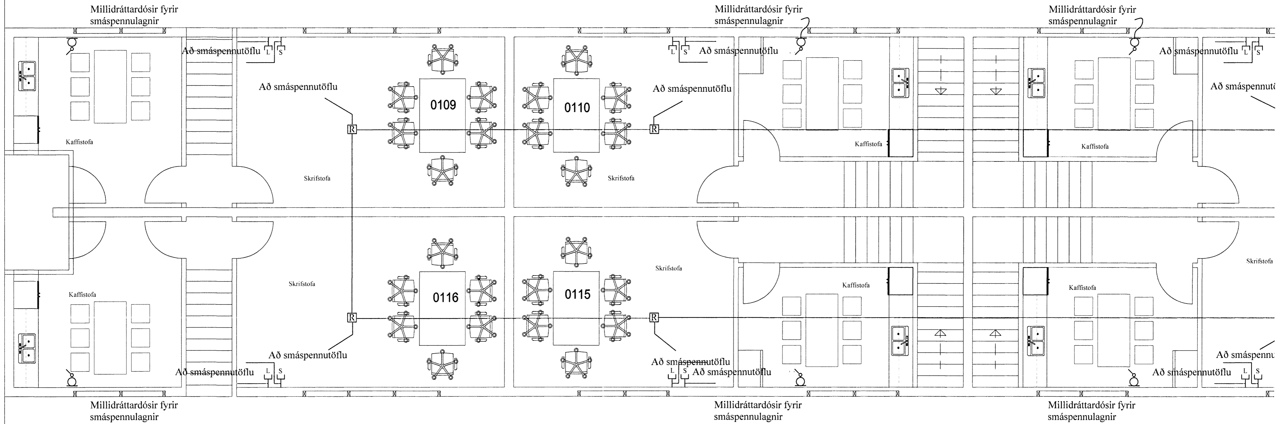
Grunnmynd Smáspennulögn 2. hæð
