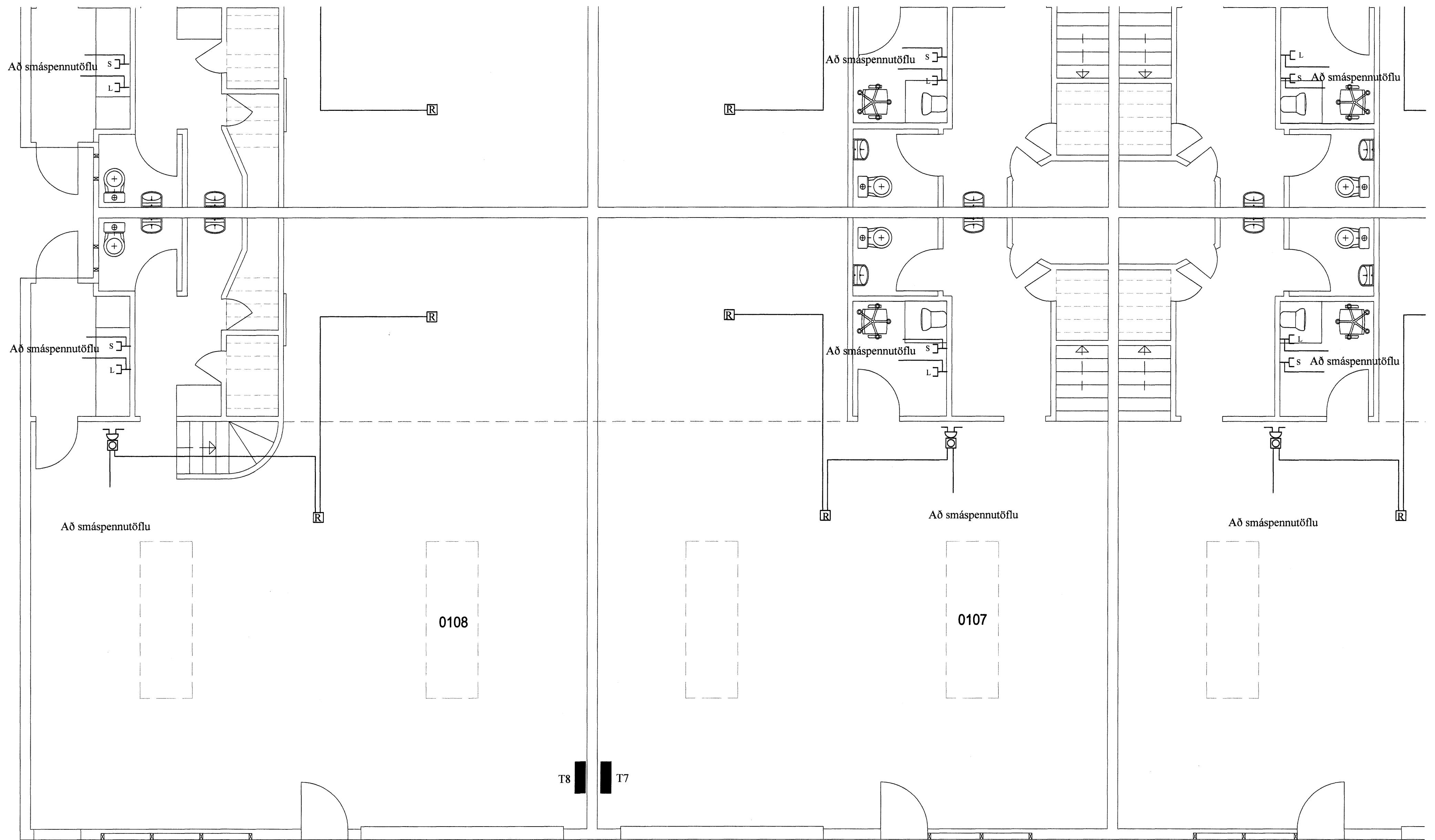
Grunnmynd Smáspennulögn 1. hæð
