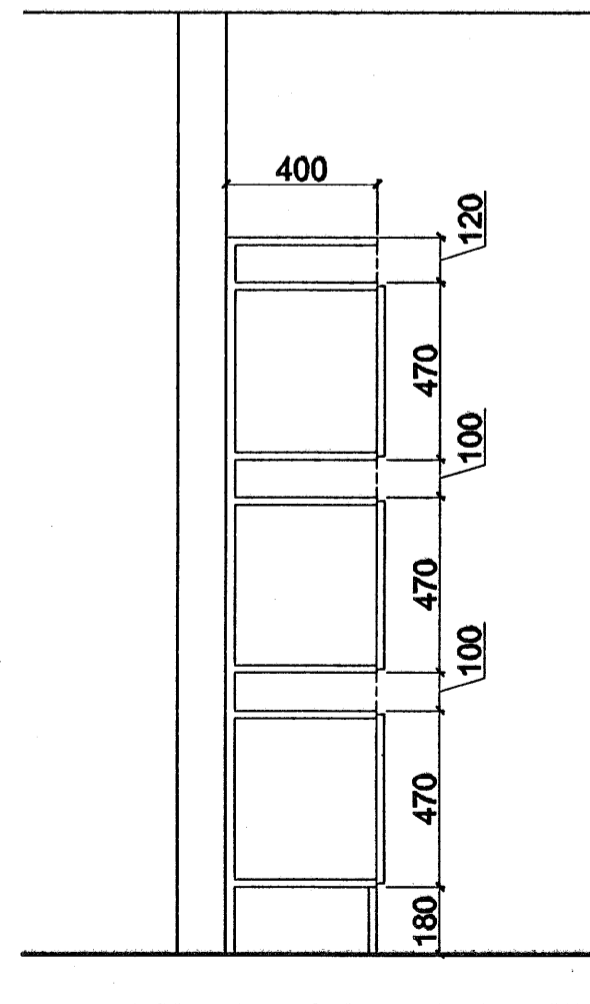
Starfsmannaskápar - sneiðing mkv. 1:20
