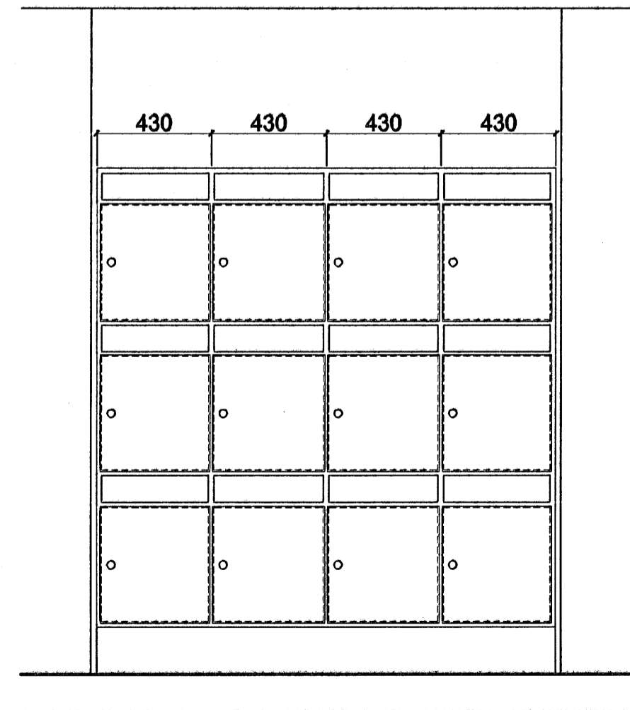
Starfsmannaskápar - ásynd mkv. 1:20
