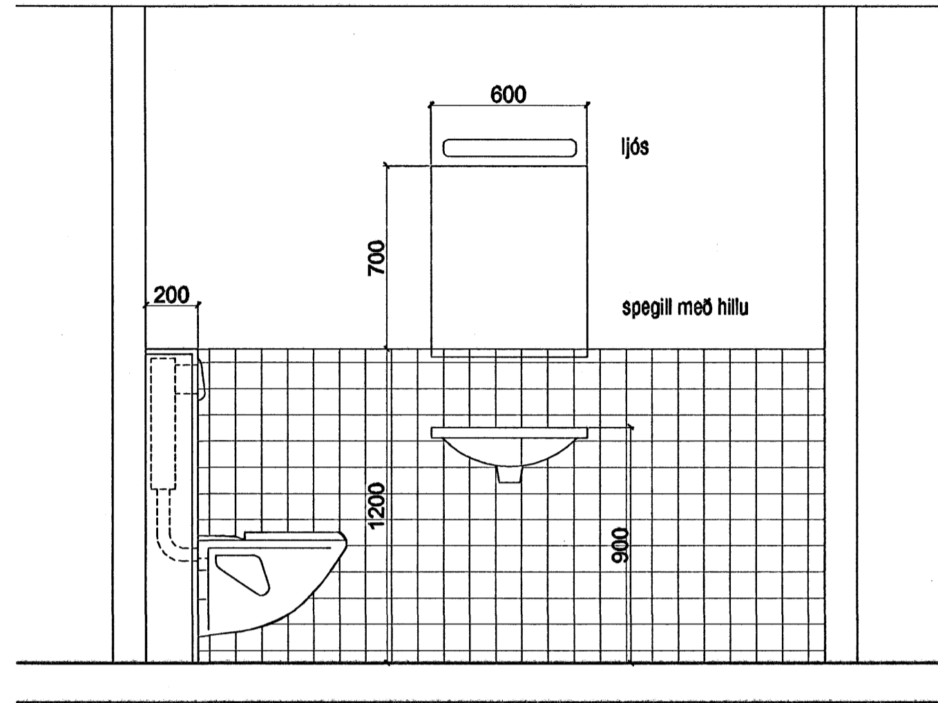
Snyrtingar - dæmigerður frágangur mkv. 1:20
