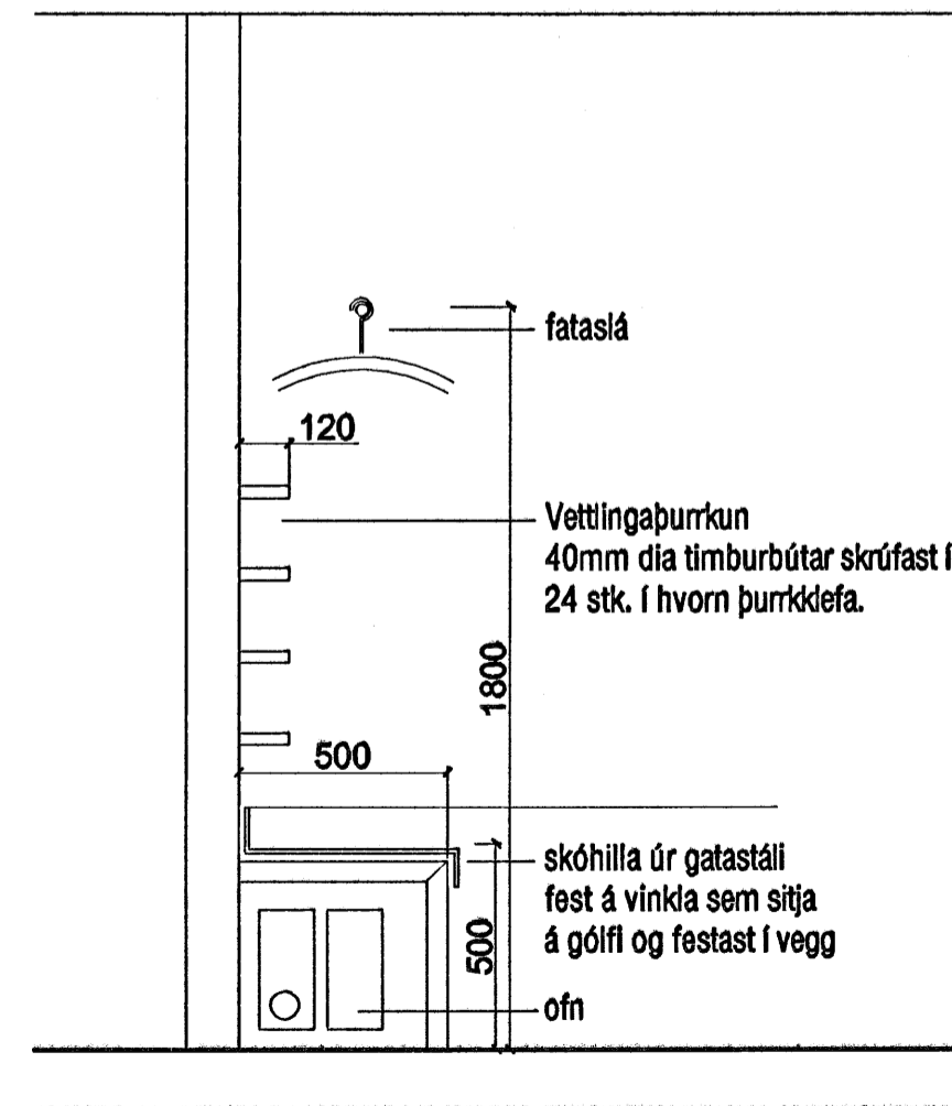
Bekkur og fataslá í þurrk-lefa mkv. 1:20
