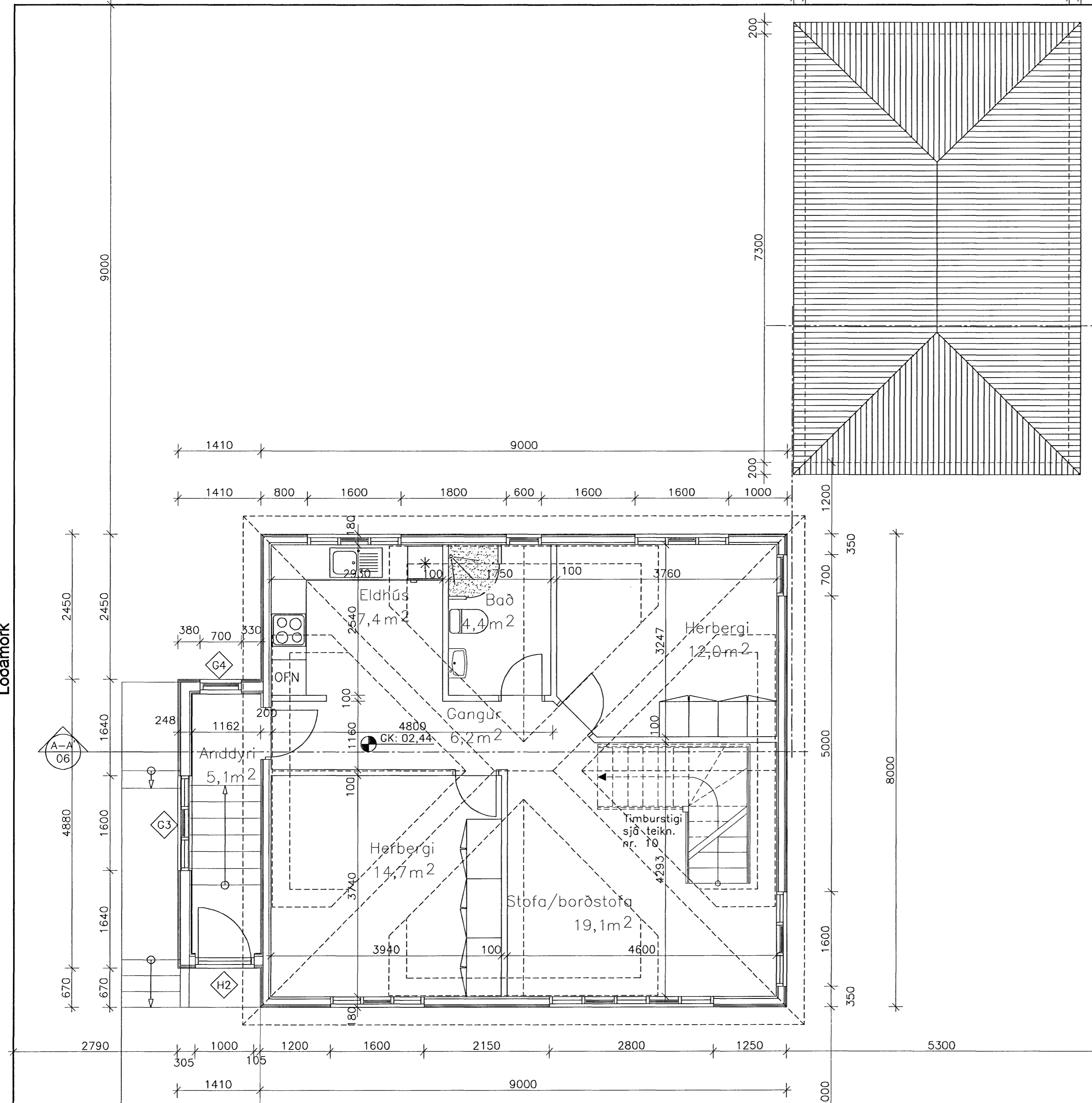
GRUNNMYND 1. HÆÐAR 1:50
