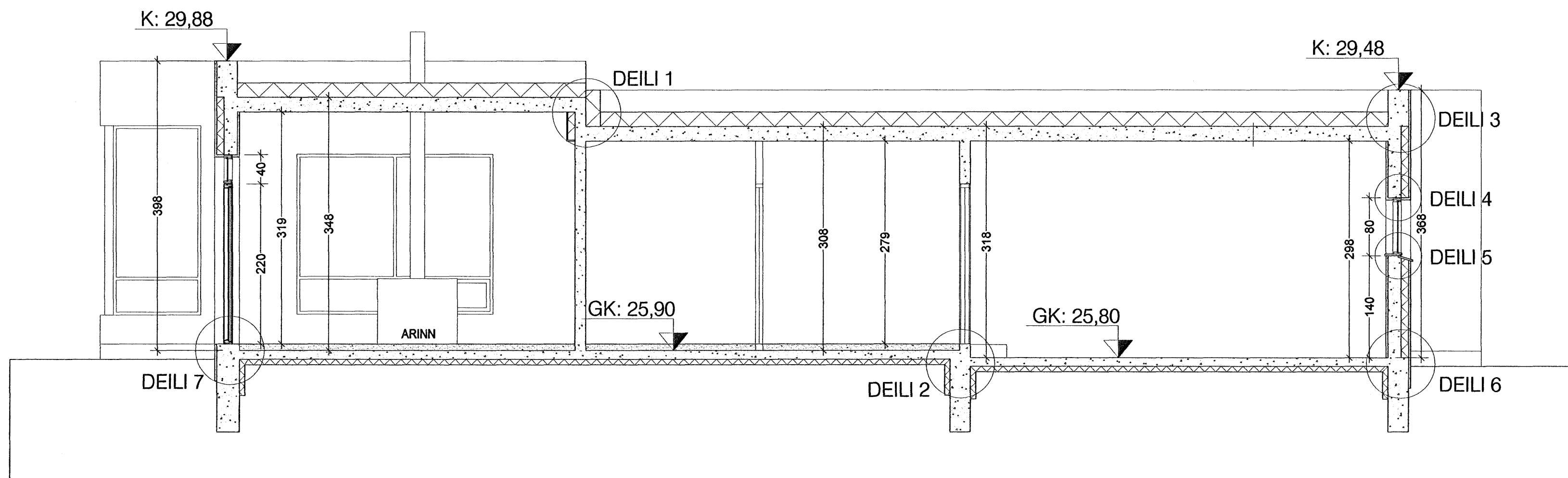
SNEIÐING A-A
