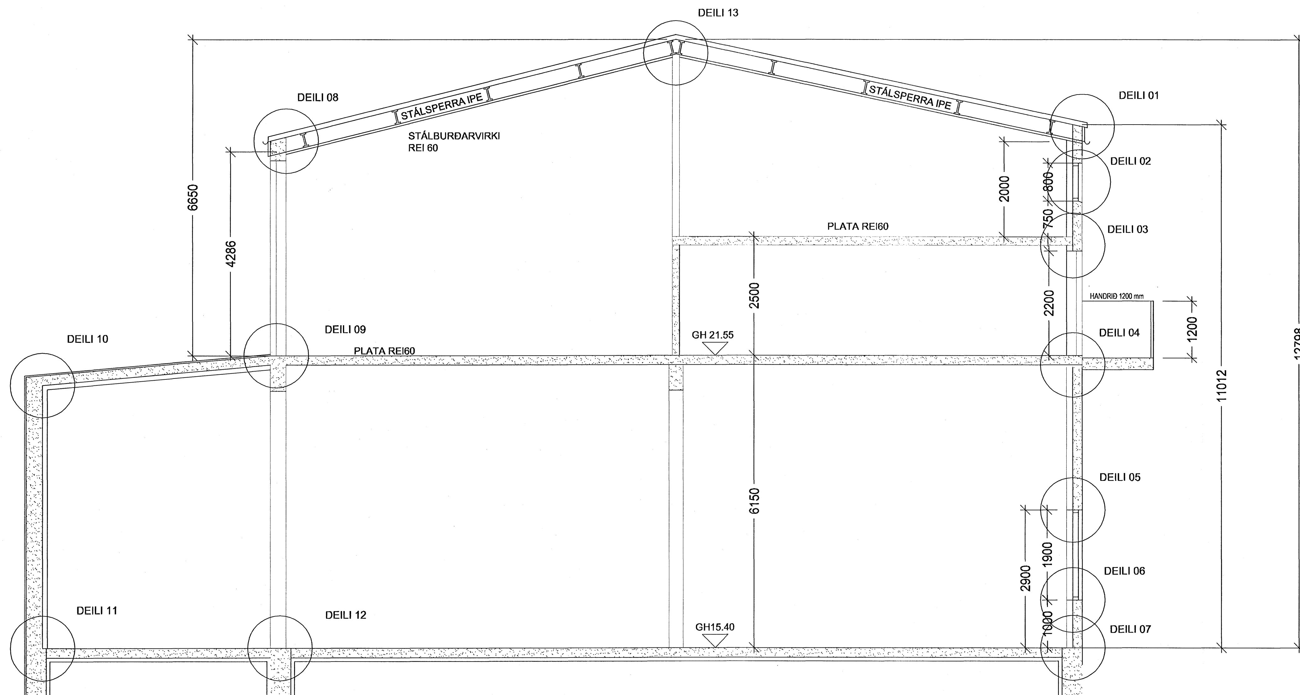
SNID A-A 1:50
