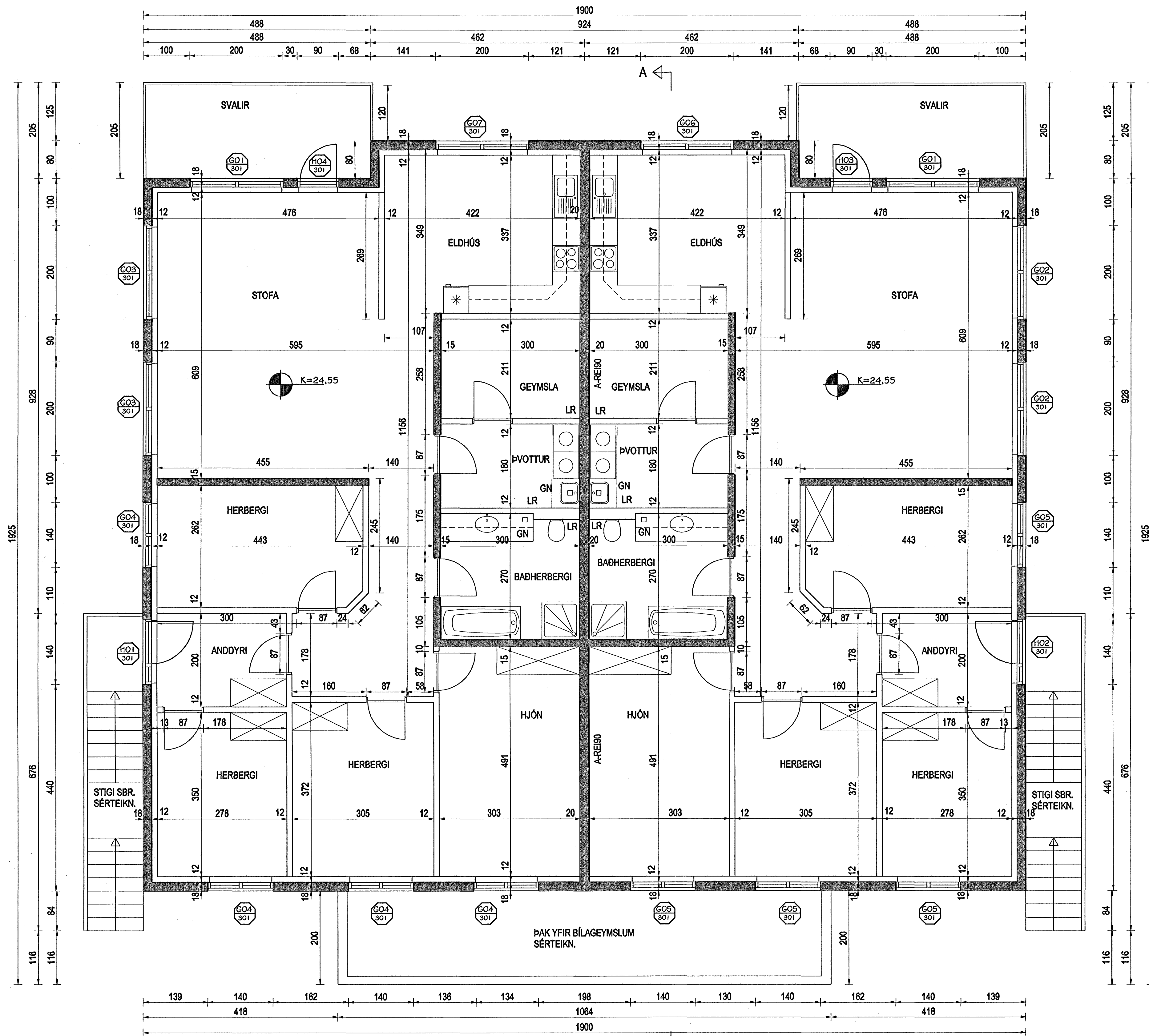
GRUNNMYND EFRI HÆÐAR MKV. 1:50
