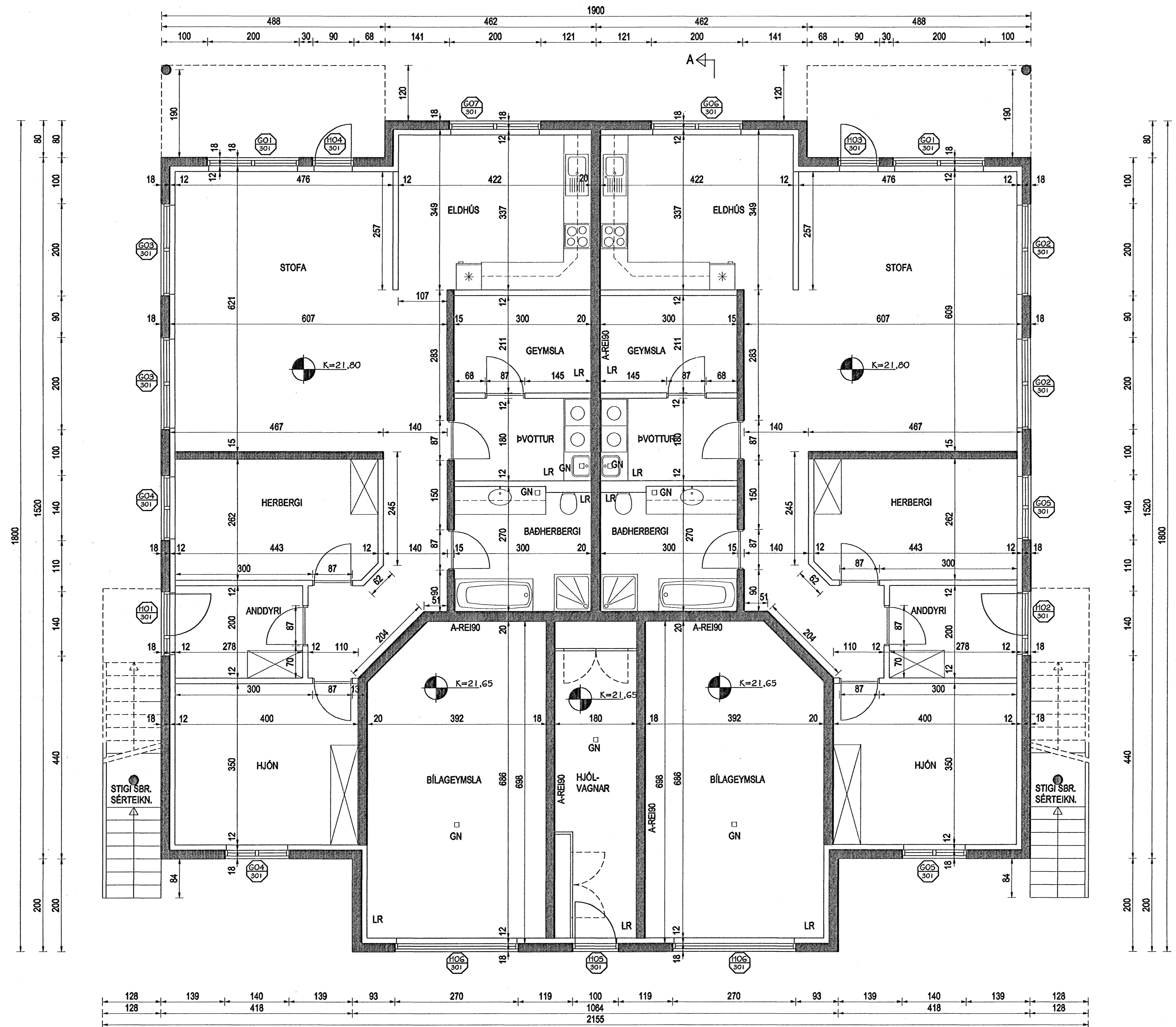
GRUNNMYND NEDRI HÆÐAR MKV. 1:50
