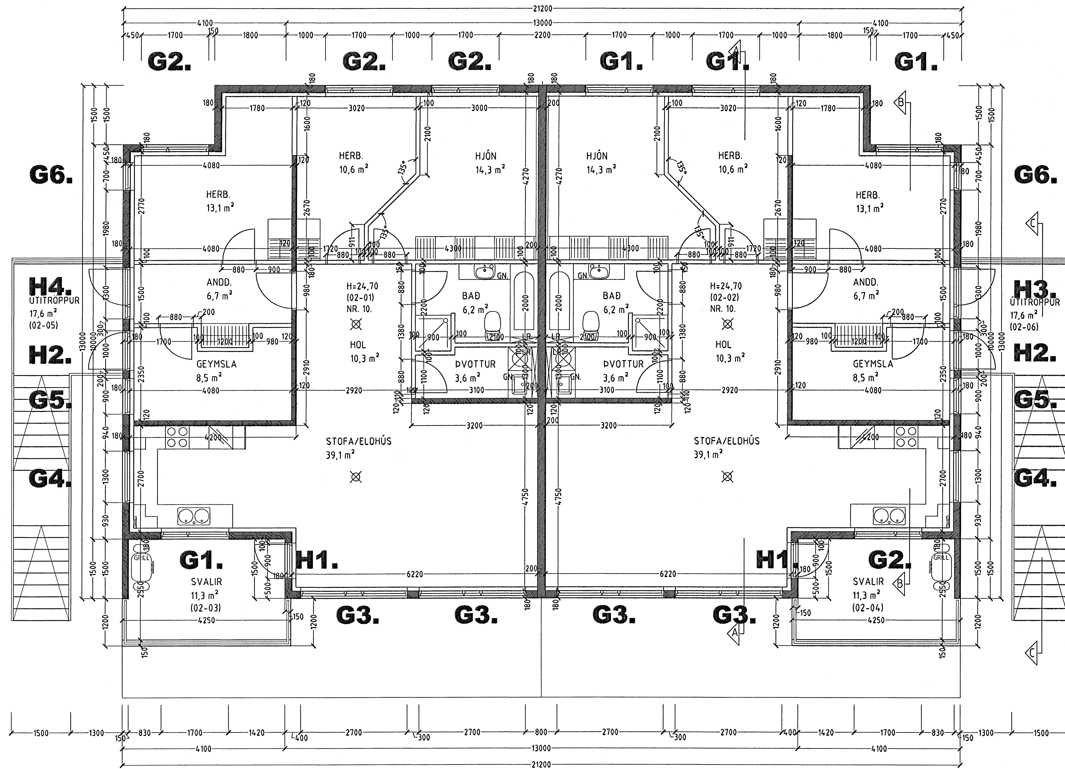
GRUNNMYND 2. HÆÐ MKV. 1:50.
