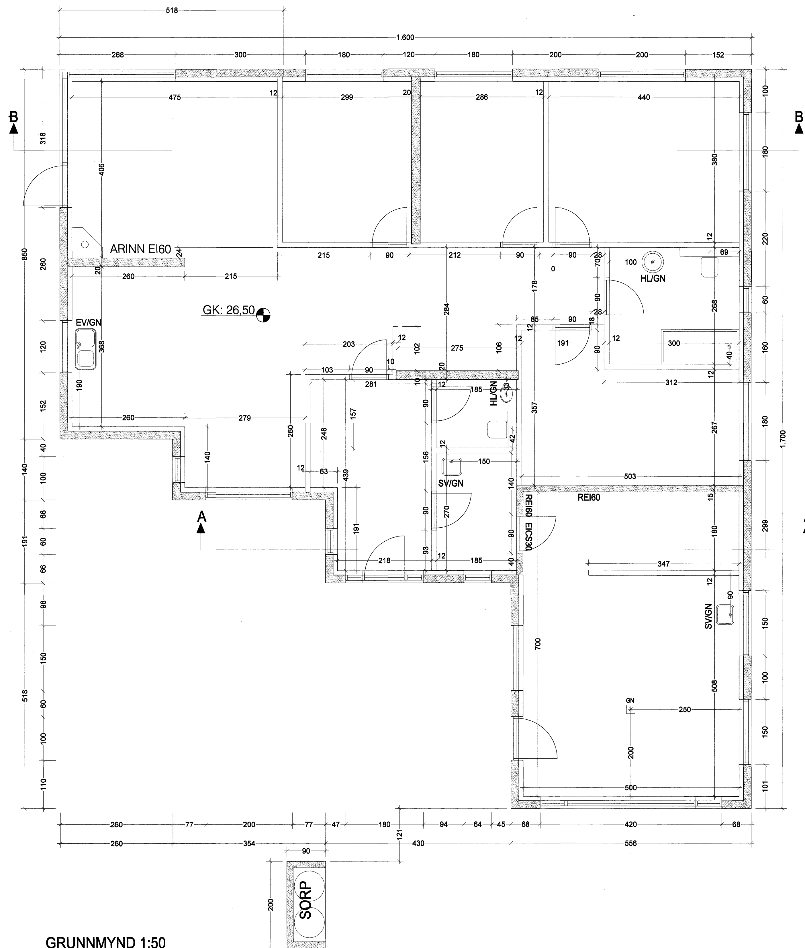
GRUNNMYND 1:50
